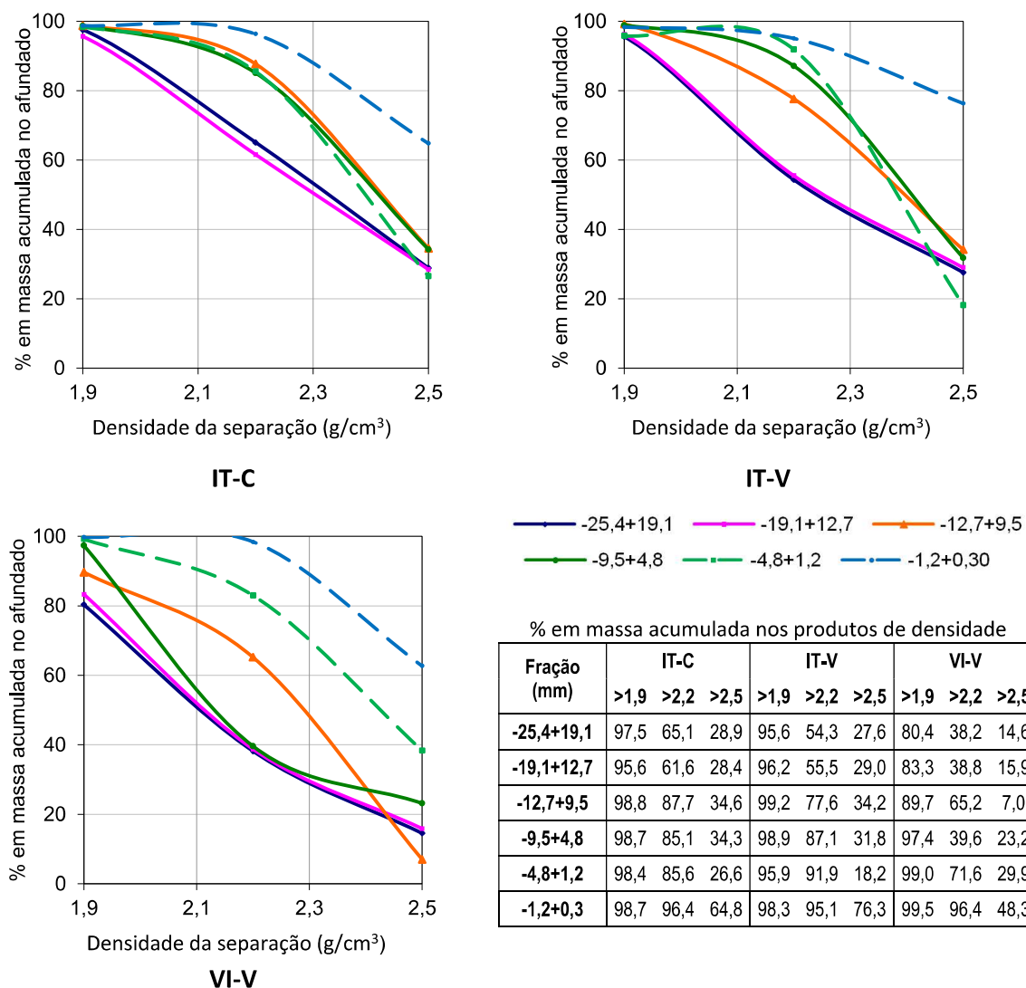
Figura 1 - Curvas de separabilidade por densidade.
