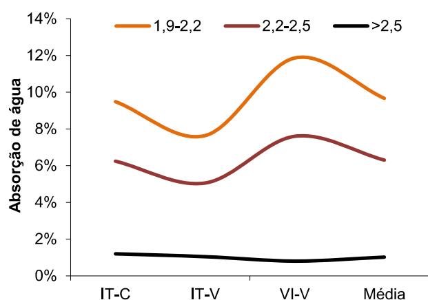
Figura 3 - Absorção de água para os diferentes produtos da separação por densidade
