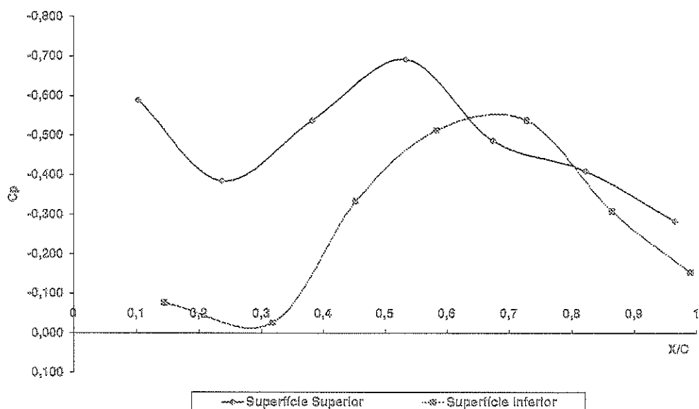
Fig.(10) – Distribuição C_p x X/C na seção central do "Nacele Pusher" 2 para ângulo de 4 graus.
