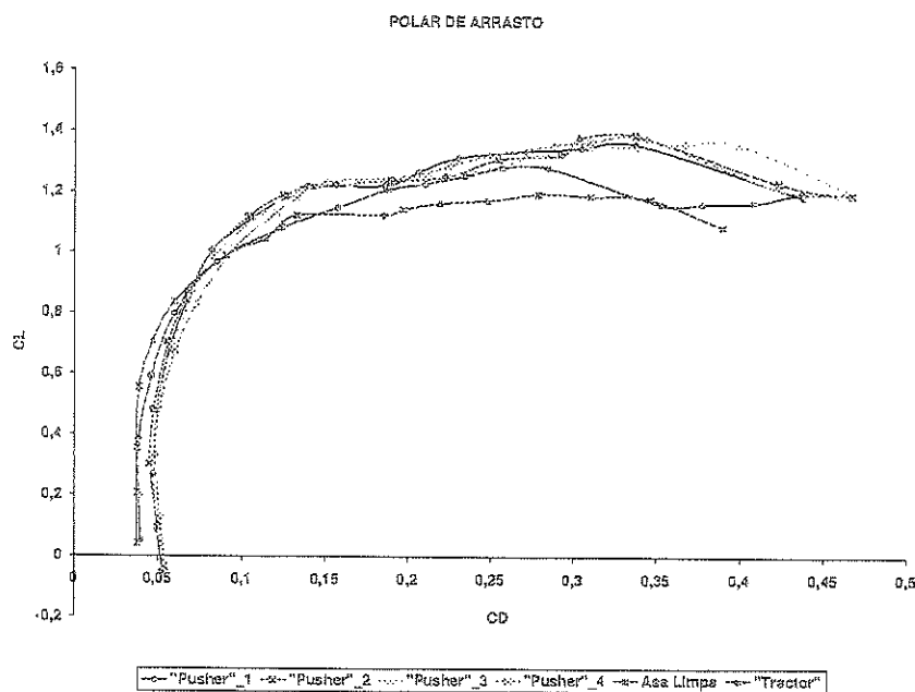
Fig.(6) – Polar de Arrasto para diferentes configurações
