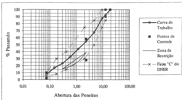
Figura 2: Curva granulométrica da mistura estudada
