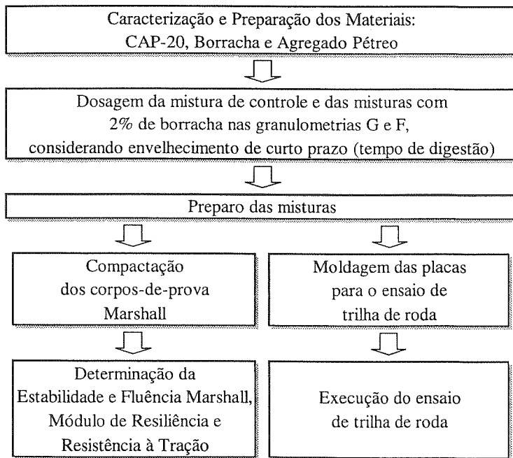
Figura 1: Diagrama de blocos do método de trabalho experimental
