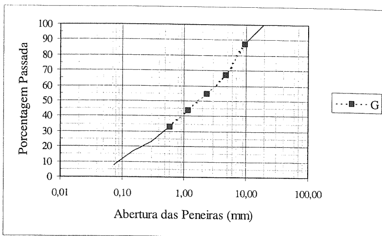
(a) Mistura com borracha na granulometria G: 9,5 mm (3/8") até 0,60 mm (#30)
