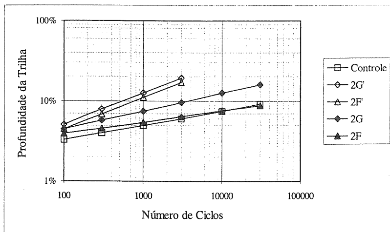
Figura 5: Resultados dos ensaios de trilha de roda
