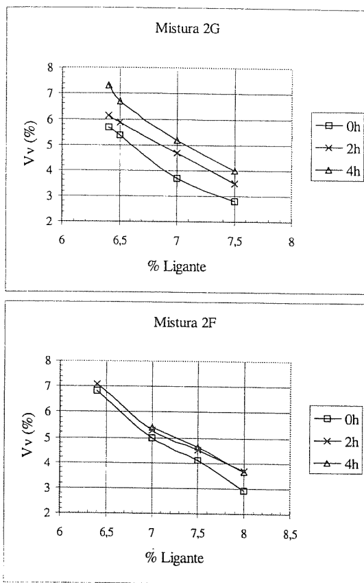
Figura 4: Efeito do envelhecimento (tempo de digestão) para as misturas com borracha
