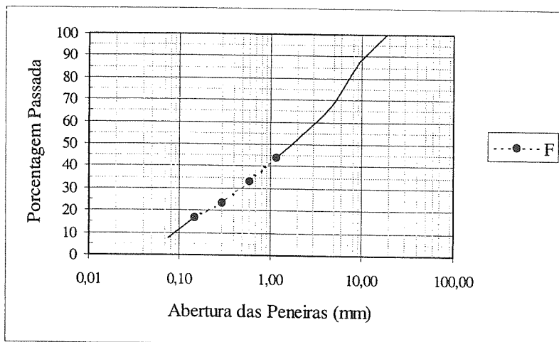
(b) Mistura com borracha na granulometria F: 1,18 mm (#16) até 0,15 mm (#100)
