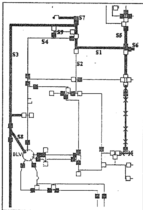
Fig. 9: Configuração após o plano de restabelecimento de energia ter sido executado
