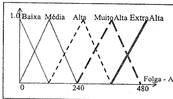
Fig. 3: Conjuntos fuzzy para folga do alimentador.
