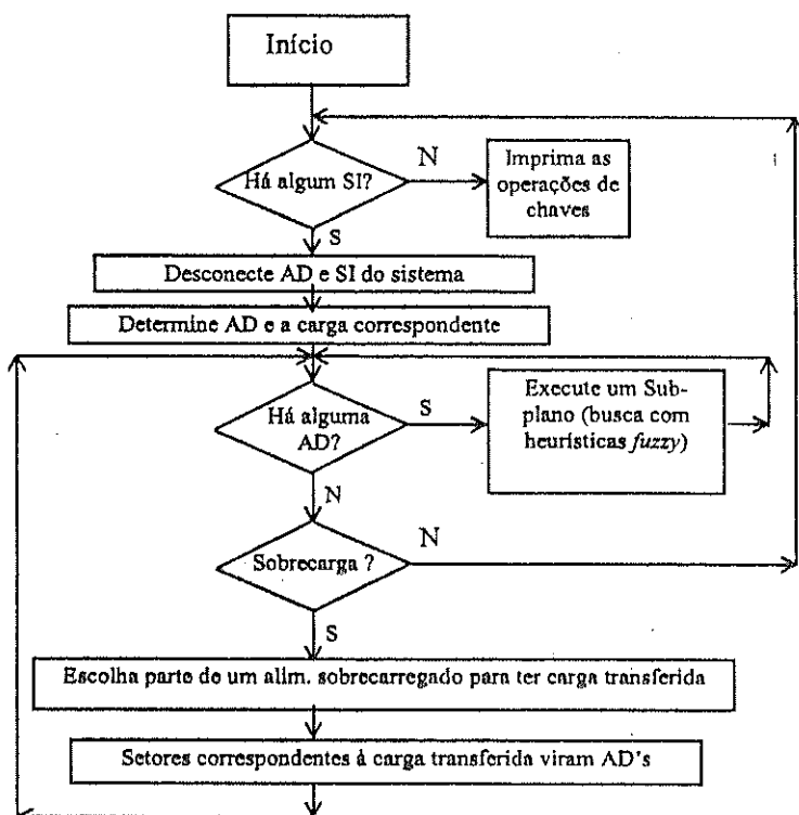
Fig. 7: Fluxograma do procedimento de restabelecimento de energia usando heurísticas fuzzy. (AD: Área Desenergizada e SI: Setor Isolado).
