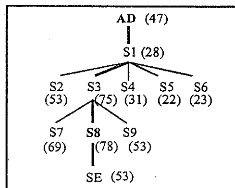
Fig. 10: Árvore de busca no estado de espaço das chaves.
