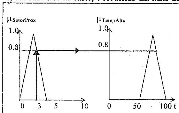
Fig. 4: Exemplo de implicação fuzzy produzida nas regras mencionadas na subseção 2.1.
