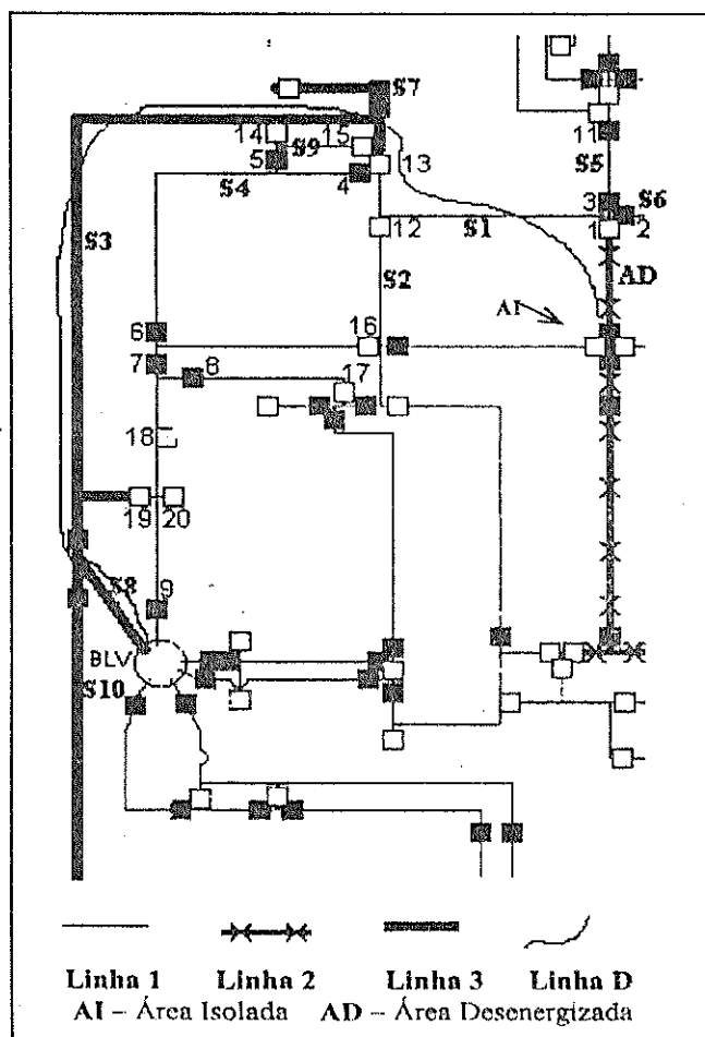
Fig. 8: Configuração antes do plano de restabelecimento de energia ter sido executado
