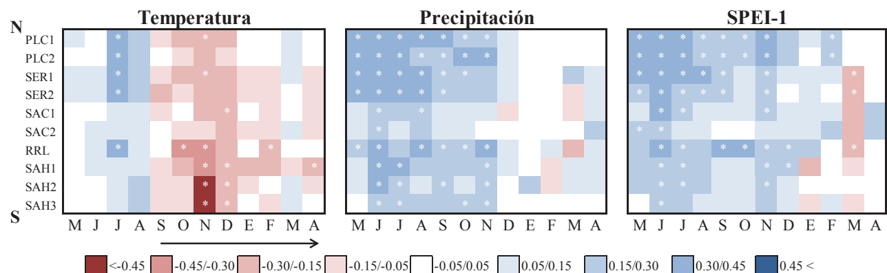
Figura 3. Análisis de correlación entre las 10 cronologías agrupadas y las variables climáticas mensuales (precipitación acumulada, temperatura media y SPEI-1), desde mayo a abril durante el periodo 1943-2014. Asteriscos indican significancia estadística al nivel de confianza de 95 % ( r = \pm 0.23 ). La flecha indica estación de activo crecimiento de los árboles. Las cronologías están ubicadas de norte a sur.
