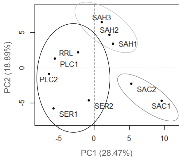
Figura 2. Posiciones relativas de las 10 cronologías de Nothofagus macrocarpa de acuerdo a los dos componentes principales para el periodo 1938-2014. Los círculos representan el agrupamiento de las poblaciones utilizando como función distancia 1-correlación de Pearson (correlación cofenética = 0,913). Fueron definidos tres grupos: (i) bosques degradados de la Cordillera de la Costa (grupo I: círculo negro), (ii) bosques poco degradados de la Cordillera de la Costa (grupo II: círculo gris); (iii) bosques poco degradados de la Cordillera de Los Andes (grupo III: círculo gris claro). Los porcentajes de los ejes indican cuánta variación de los datos fue explicada por las componentes principales.
