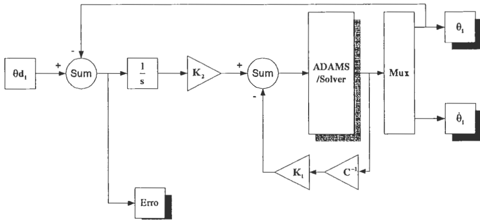
Figura 3 - Sistema de Controle Seguidor.
