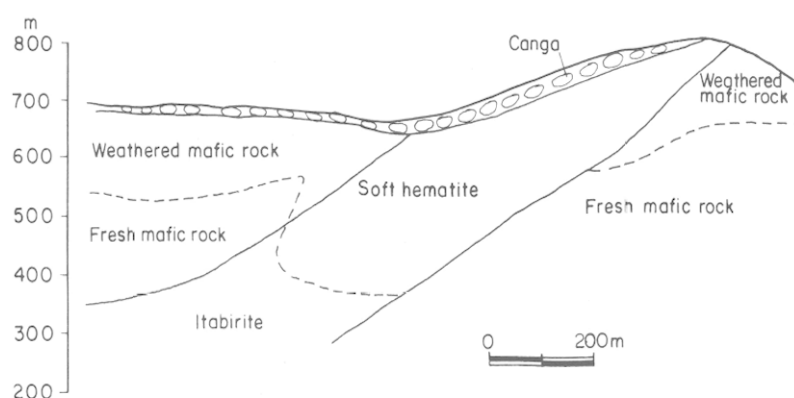
Fig. 9 — Cross section of Carajas iron deposit. Coupe du gisement de fer de Carajas.
