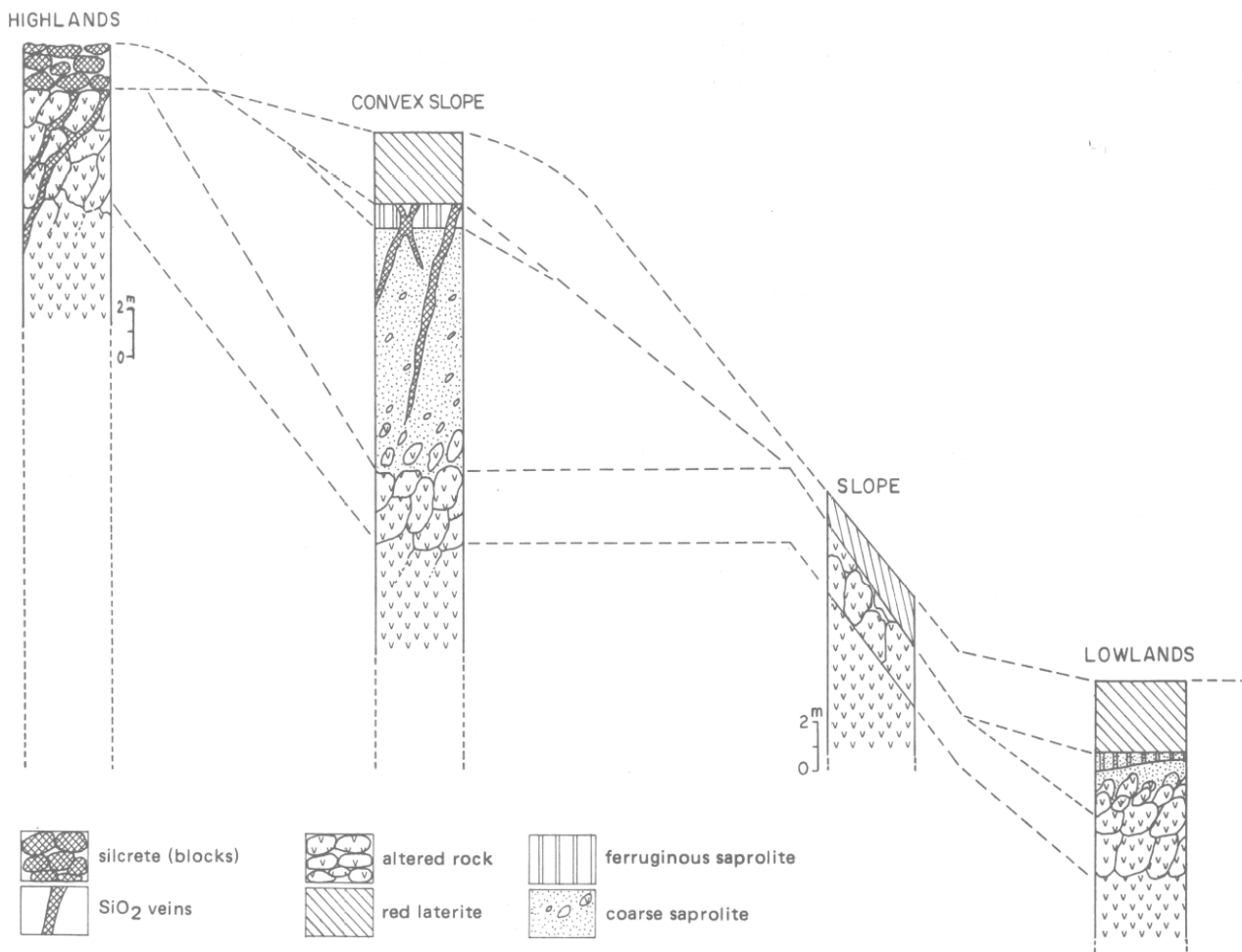
Fig. 13 — Ultramafic rocks alteration profiles morphological characteristics in highlands, slopes and lowlands in Central Brazil. Caractéristiques morphologiques de profils d'altération de roches ultrabasiques en zones hautes, sur les versants, et en zones basses, dans le Brésil central.
