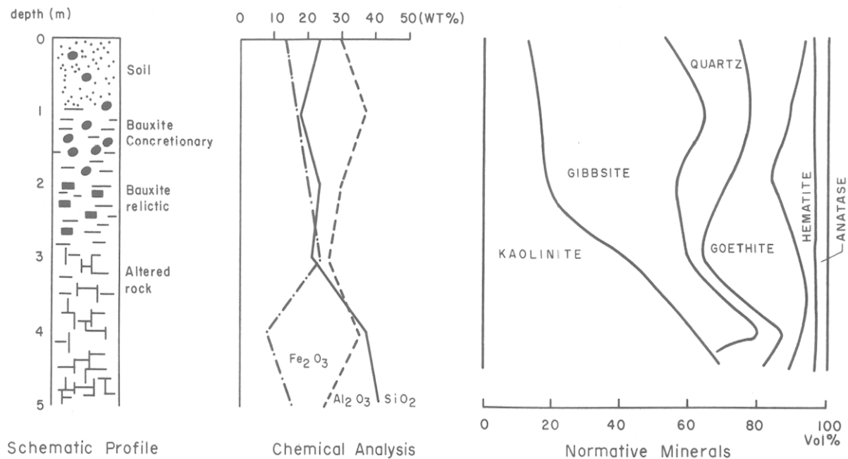
Fig. 7 — Chemical and mineralogical composition along a typical bauxite profile, Mirai (Cataguases). Variation de composition chimique et minéralogique le long d'un profil bauxitique typique, Mirai (Cataguases).
