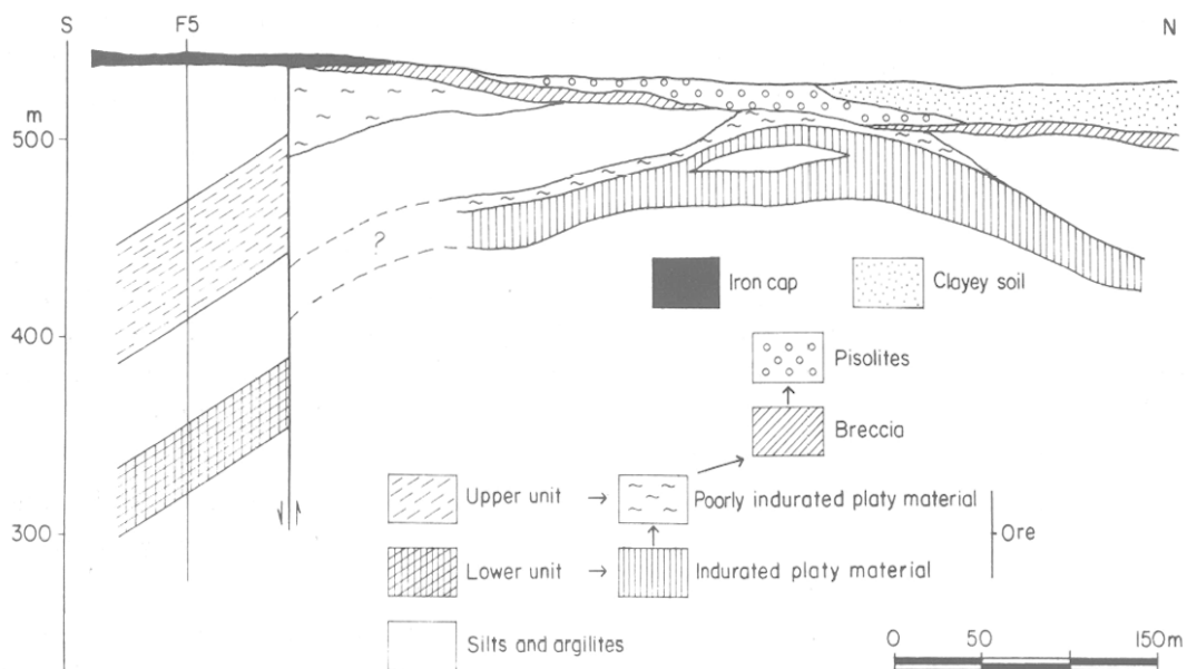
Fig. 11 — Schematic cross-section of the manganeseiferous Azul deposit, Serra dos Carajas. Coupe schématique du gisement de manganèse d'Azul, Serra de Carajas.
