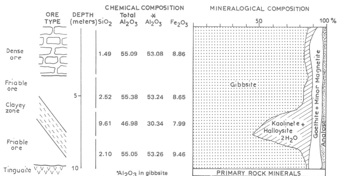
Fig. 4 — Chemical and mineralogical composition along the bauxitic ridge alteration profiles, Poços de Caldas (after ALMEIDA, 1977). Variation de composition chimique et minéralogique le long d'un profil d'altération bauxitique de versants en secteur montagneux, Poços de Caldas (d'après ALMEIDA, 1977).
