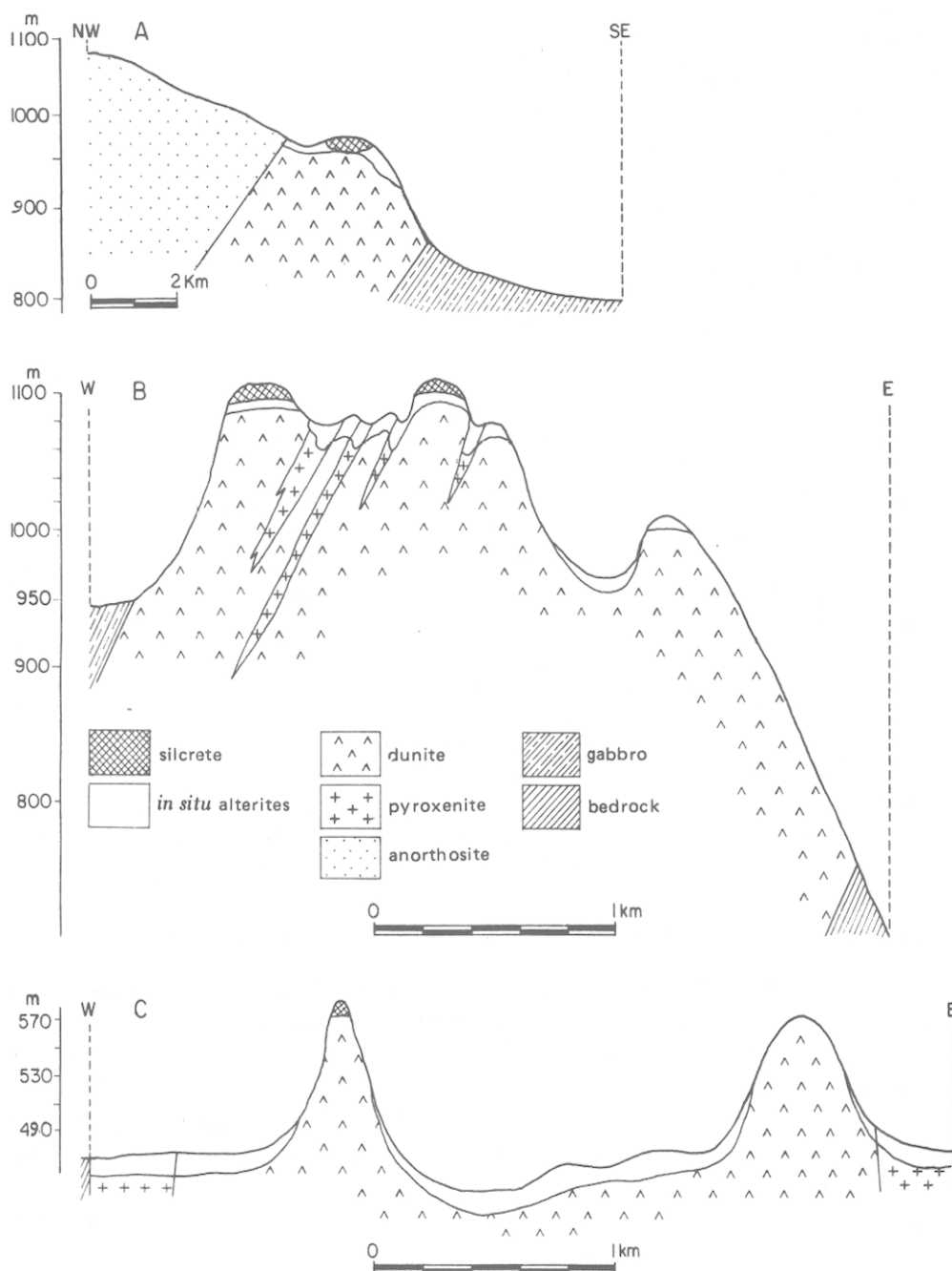
Fig. 12 — Cross-sections of nickeliferous deposits in Central Brazil : A, Barro Alto, central part ; B, Niquelandia, southern part ; C, Santa Fé. Coupes de divers gisements nickélifères du Brésil central : A, Barro Alto, partie centrale ; B, Niquelandia, partie Sud ; C, Santa Fé.
