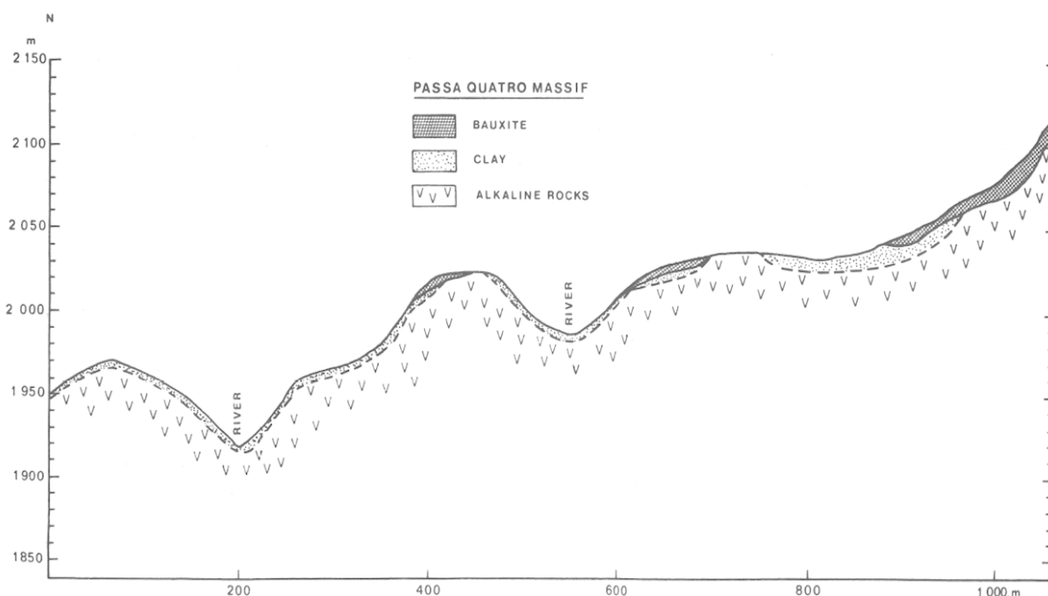
Fig. 6 — Cross-section of high plateau bauxitic deposit, Passa Quatro alkaline massif. Coupe à travers un gisement bauxitique de hauts-plateaux, massif alcalin de Passa Quatro.
