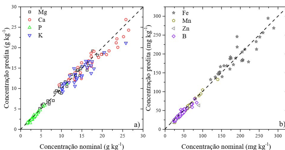
Figura 3. Comparação da concentração de nutrientes em folhas de soja predita pelo método CF-LIBS com a técnica de AAS, para os: a) macros e b) micronutrientes.
