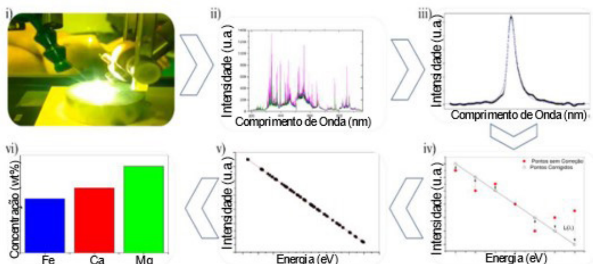
Figura 2. Fluxograma mostrando: i) medida LIBS, ii) tratamento dos espectros, iii) correção da linha de base e cálculo das áreas das emissões dos elementos, iv) calibração pelo OPC, v) cálculo dos parâmetros do plasma, vi) quantificação dos elementos interesse.
