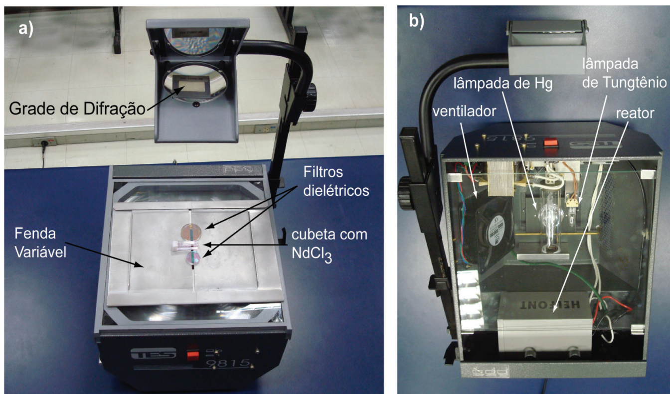
Figura 1S. a) Fotografia mostrando o retroprojektor em uma configuração típica de observação dos espectros de transmissão. b) Figura do interior do retroprojektor, enfatizando as modificações realizadas
