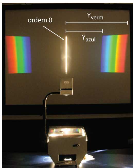
Figura 3. Fotografia mostrando a decomposição da luz branca (lâmpada de tungstênio original do retroprojektor). Distância L = 3 m e grade de difração de 600 linhas/mm. A curvatura apresentada pelo padrão deve-se à aberração esférica na lente de focalização do retroprojektor
