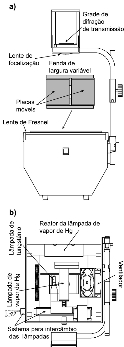
Figura 1. a) Desenho esquemático da vista lateral do retroprojektor com a fenda de largura variável evidenciada. b) Corte transversal (visto de cima) do interior do retroprojektor. (Ver fotografia do retroprojektor modificado na Figura 1S do material suplementar)
