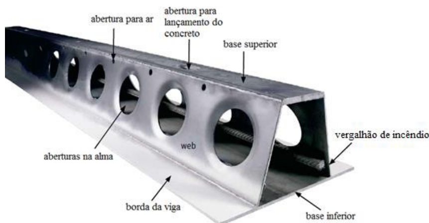
Figura 3. Deltabeam® [6]
