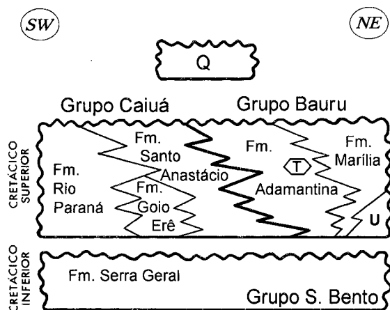
Figura 5.- Relaciones entre las unidades litoestratigráficas en la Cuenca Bauru. Leyenda: U: Fm. Uberaba, T: Analcimitas Taiúva y Q: sedimentos cenozoicos.
