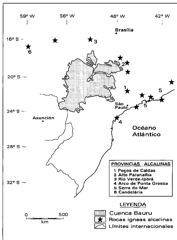
Figura 3.- Altos estructurales y áreas de magmatismo alcalino en el Cretácico Superior, en los márgenes de la Cuenca Bauru. Las "Provincias alcalinas" fueron definidas por Almeida (1983).
