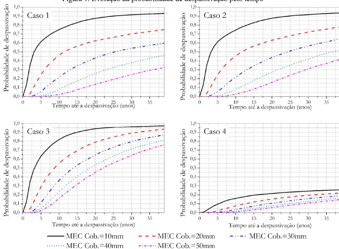
Figura 10. Evolução da probabilidade de despassivação pelo tempo
