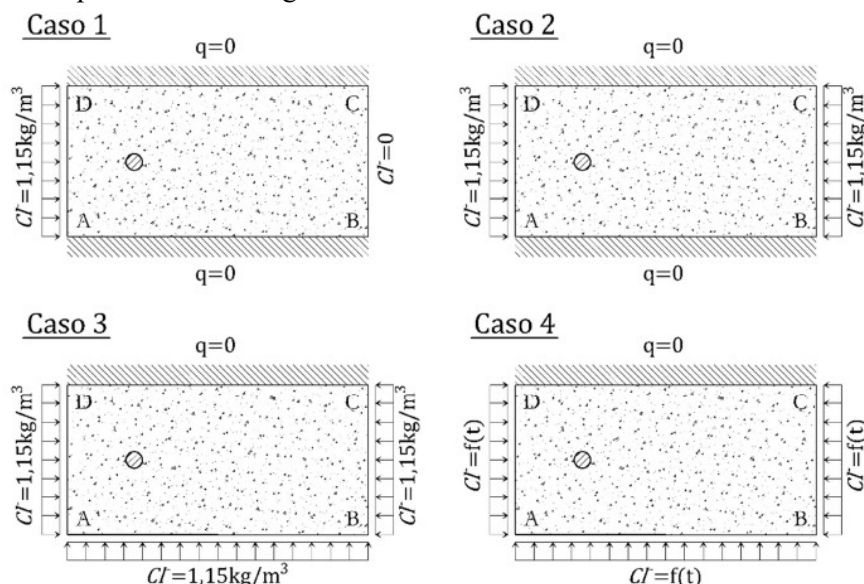
Figura 5. Condições de contorno do exemplo 1
