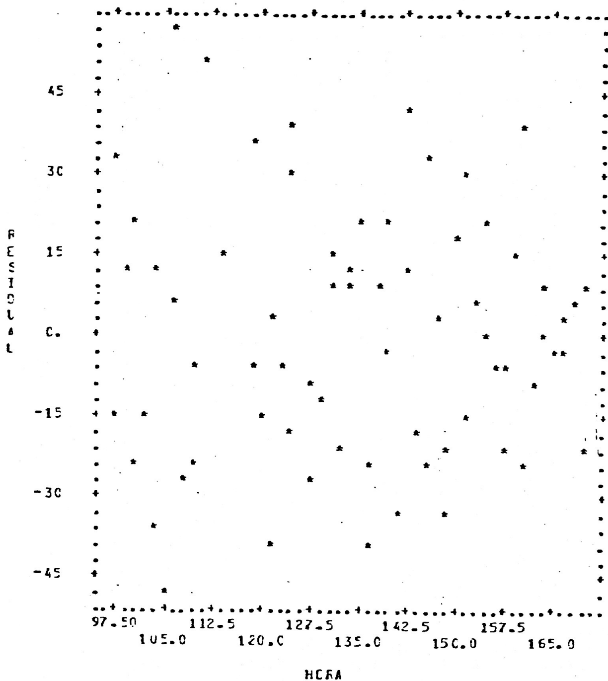
GRAFICO A4 - Resíduos da regressão pela hora.
