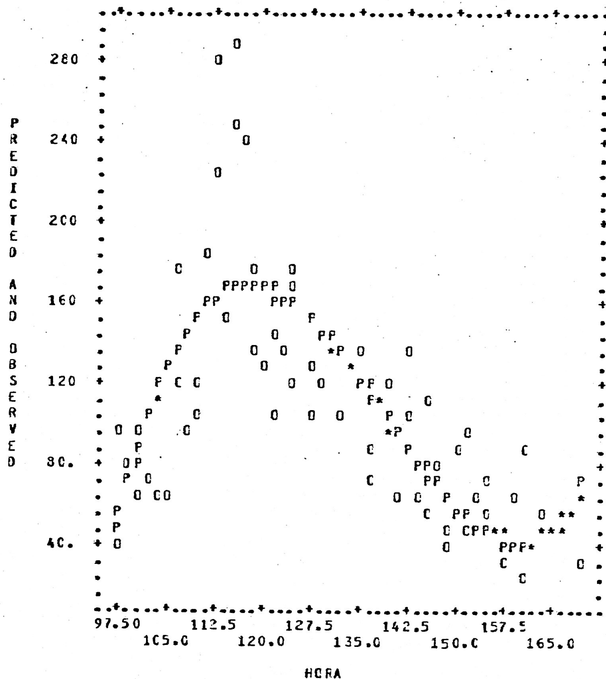
GRAFICO A1 - Valores observados e previstos em função da hora.
