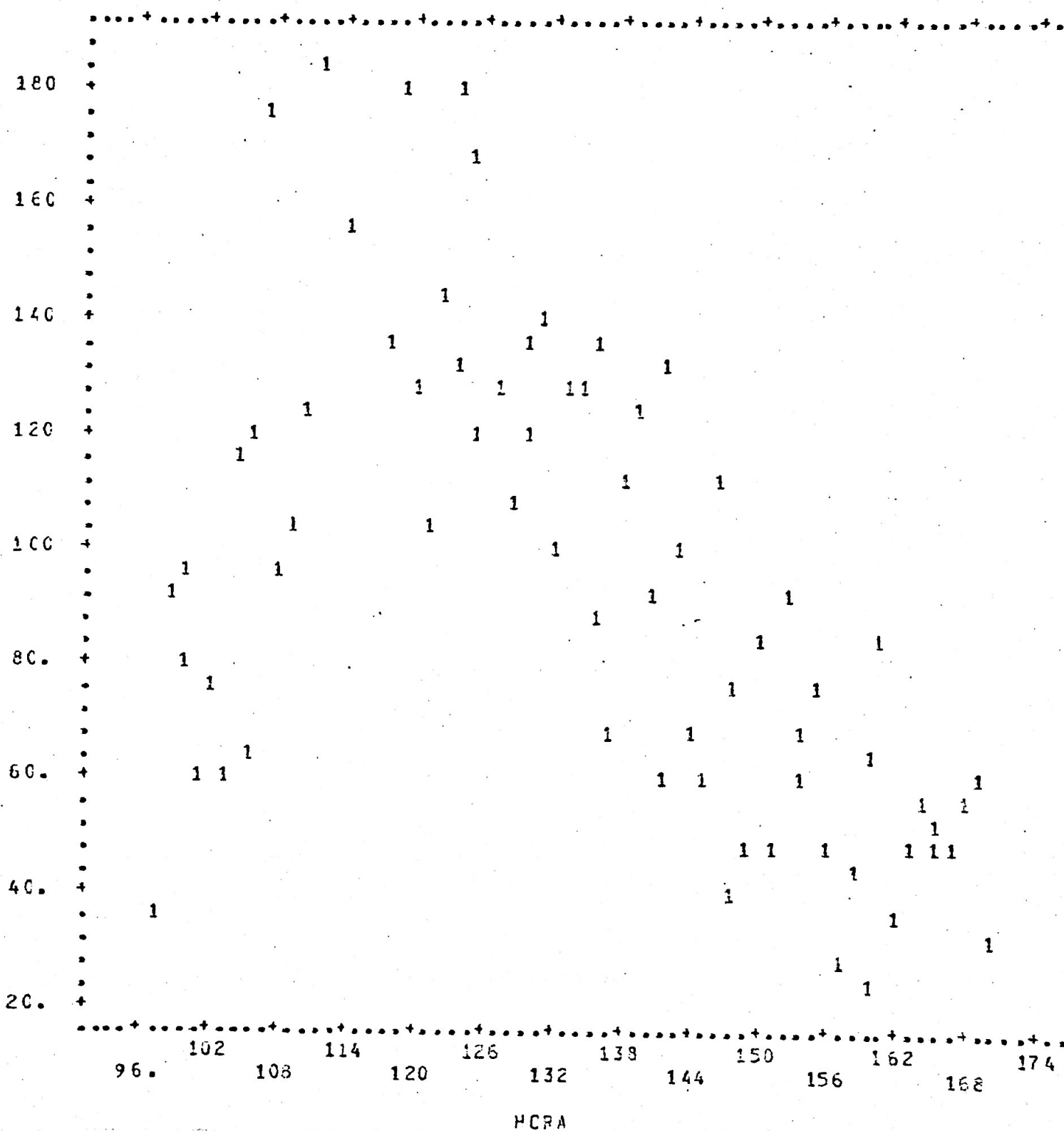
GRAFICO 1 - Diagrama de dispersão (área x hora)
