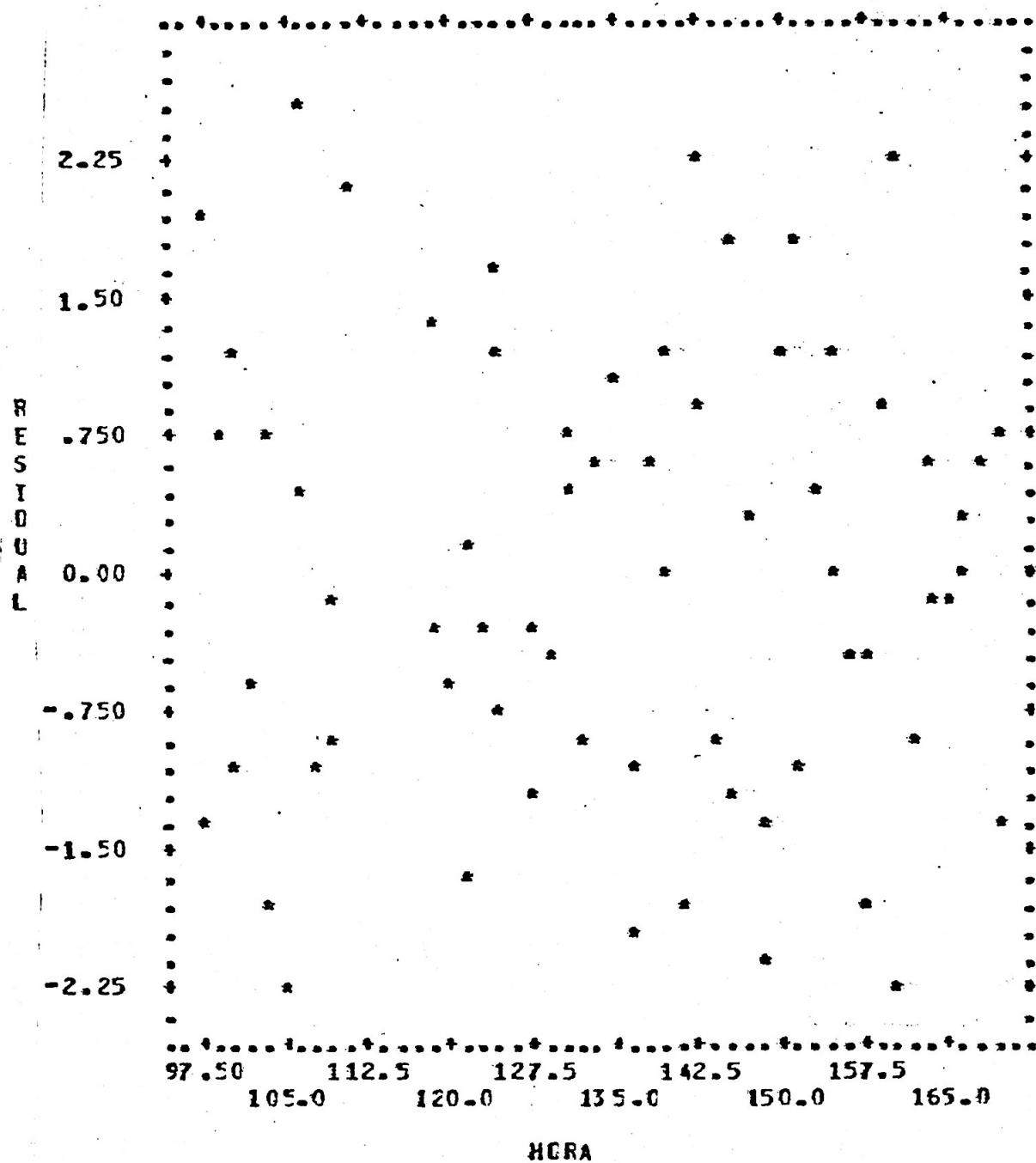
GRAFICO 2 - Resíduos da regressão em função da hora.
