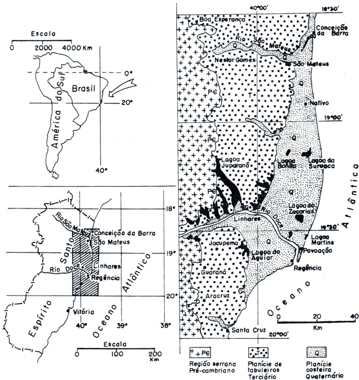
Fig. 1 - Situação geográfica e características geomorfológicas da planície costeira do rio Doce.
