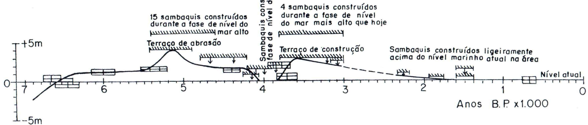
b) Região de Cananéia-Iguape (SP). SUGUIO e MARTIN (1978).
