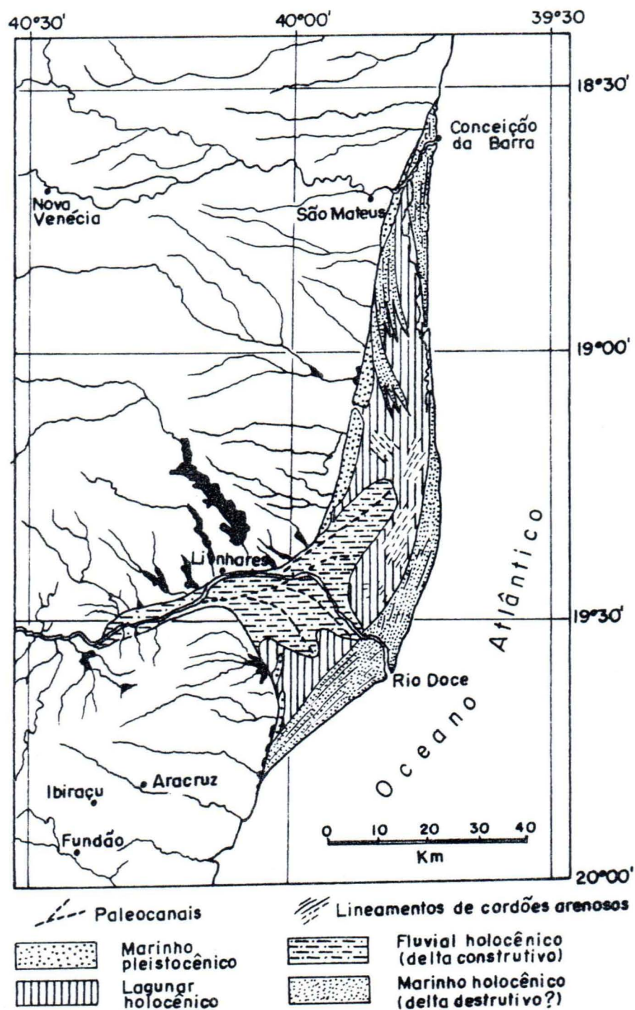
Fig. 3 – Depósitos sedimentares quaternários da planície costeira do rio Doce.
