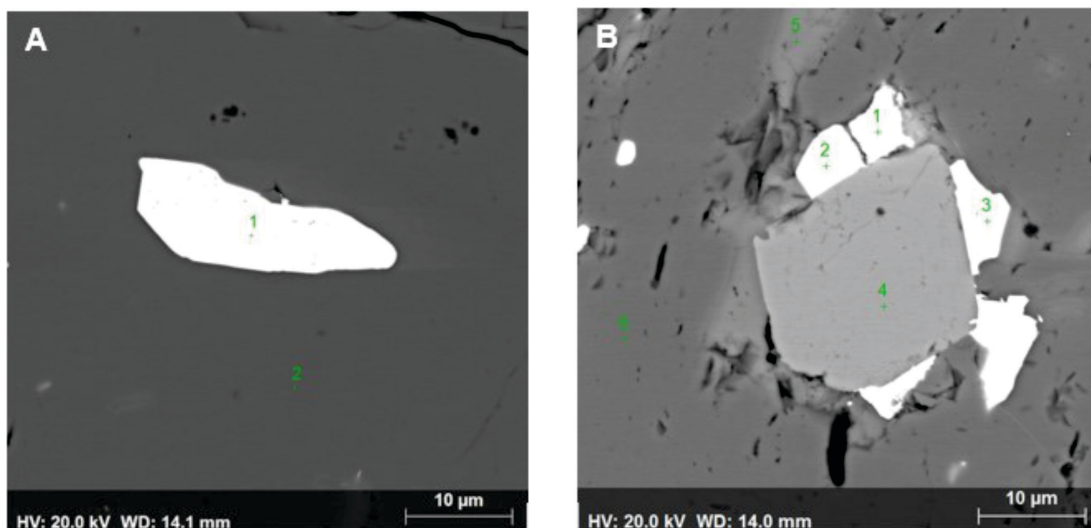
Figura 11. A: Ouro (1) potencialmente não extraído, incluído em pirita (2). B: Ouro potencialmente não extraído (1, 2 e 3) entre grãos de arsenopirita (4), calcopirita (5) e pirita (6).
