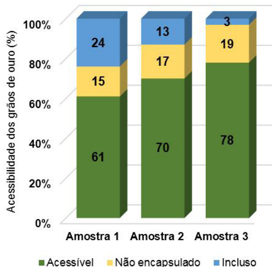
Figura 9. Acessibilidade dos grãos de ouro.
