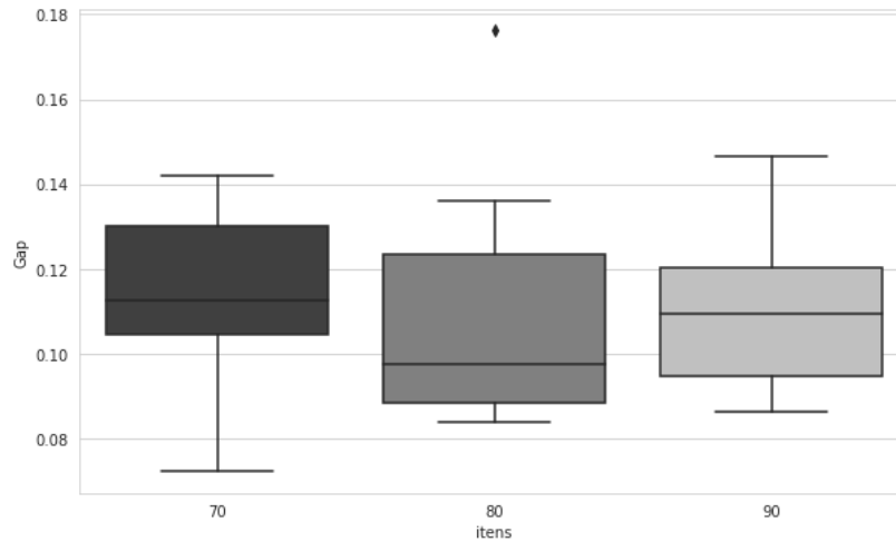
Figura 1: Box plot do Gap entre o limitante inferior e superior obtido pelo Gurobi com tempo limite de 900 para instâncias com 70, 80 e 90 itens.
