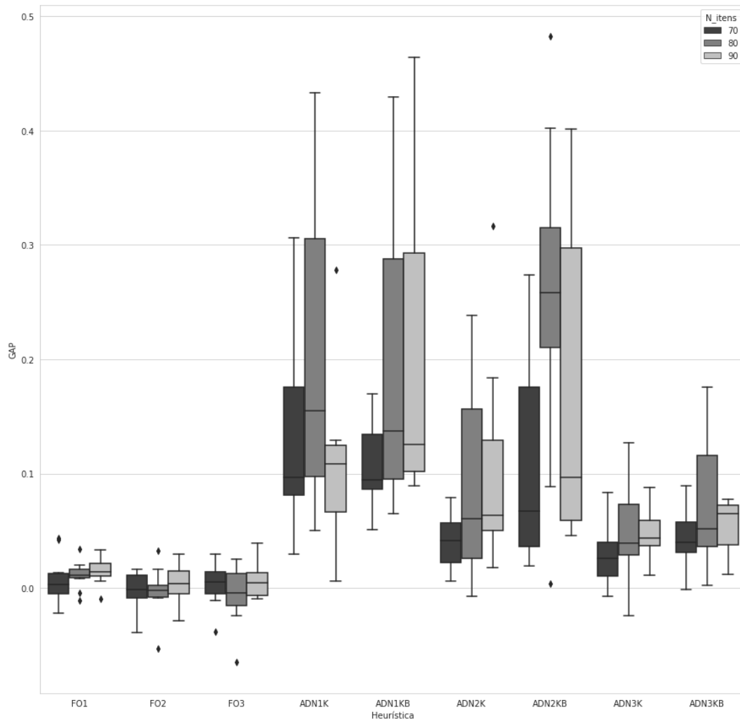
Figura 2: Boxplot do GAP de todas das heurísticas FO e ADN para instâncias com 70, 80 e 90 itens.
