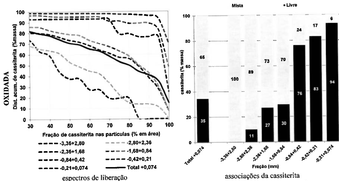
Figura 2. Curvas de espectro de liberação (em área) e formas de associação da cassiterita.
