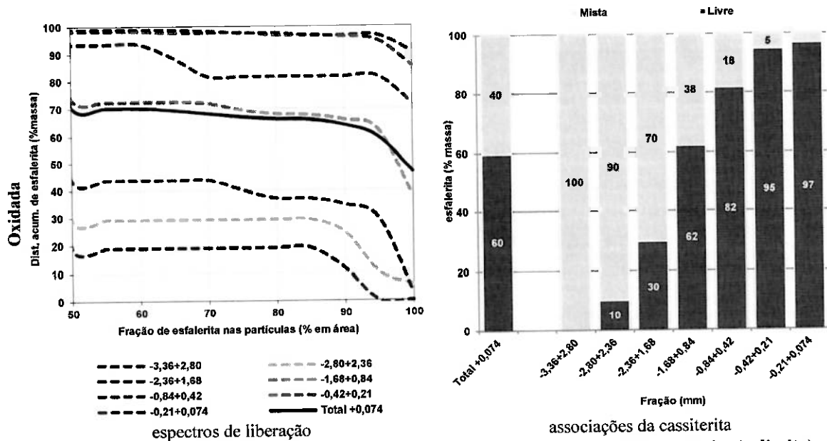
Figura 3. Curvas de espectro de liberação (à esquerda) e formas de associação da esfalerita (à direita).
