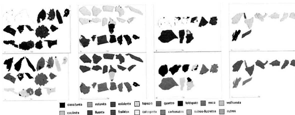
Figura 1. Fotomicrografias das partículas extraídas das imagens de elétrons retroespalhados (BSE; acima) para classificação e processamento no MLA (em falsa cor). As partículas classificadas no MLA ilustram a distinção entre cassiterita e esfalerita e os principais minerais presentes
