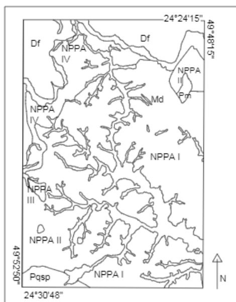
Figura 2 - Mapa geológico da área de estudo (adaptado de Guimarães, 1995): Ca (aluviões); Md (diabásio); Df (Fm. Furnas); Granito Joaquim Murtinho: NPPAV (granitos inequigranulares a porfíricos) + NPPA IV (álcali-feldspato granitos); NPPA III (granitoides inequigranulares a porfíricos); NPPA II (monzogranitos a granodioritos); NPPA I (monzogranitos a granodioritos); Pm (milonitos); Pqsp (Quartzito Serra das Pedras).
