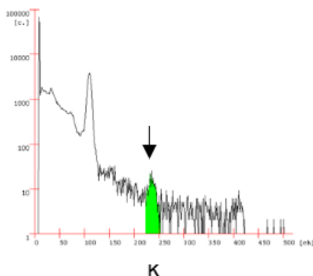
Figura 6 – Espectro do K sobre rocha alterada (GJM).
