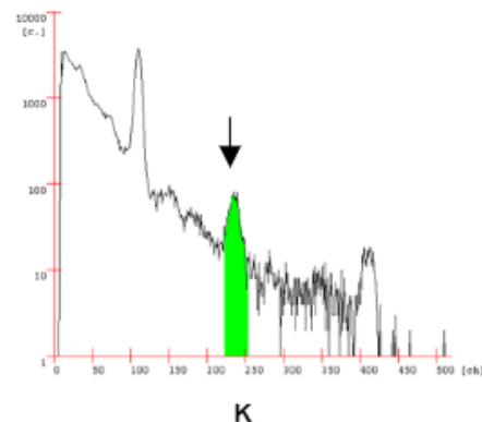
Figura 5 – Espectro do K sobre rocha fresca (GJM).
