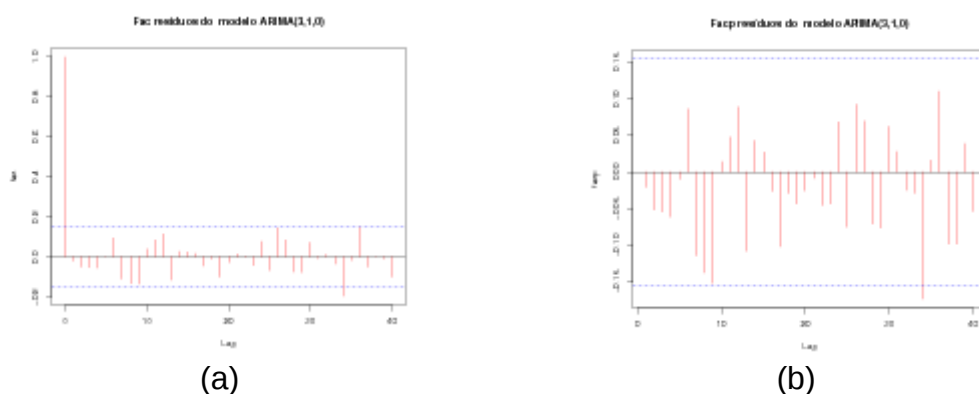
FIGURA 5: Representação gráfica das funções de autocorrelação (a) e função de autocorrelação parcial (b) dos resíduos do modelo ARIMA(3,1,0).
