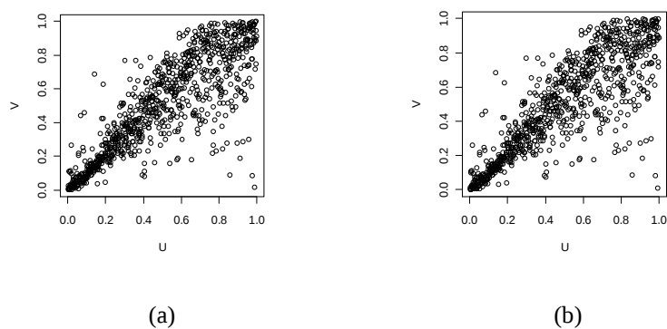
Figura 6 – Considerando o lucro líquido (X, em US$ milhões) e a margem sobre as vendas (Y, em %), temos os gráficos dos postos normalizados dos dados com outliers em (a) e sem 6 outliers em (b).
