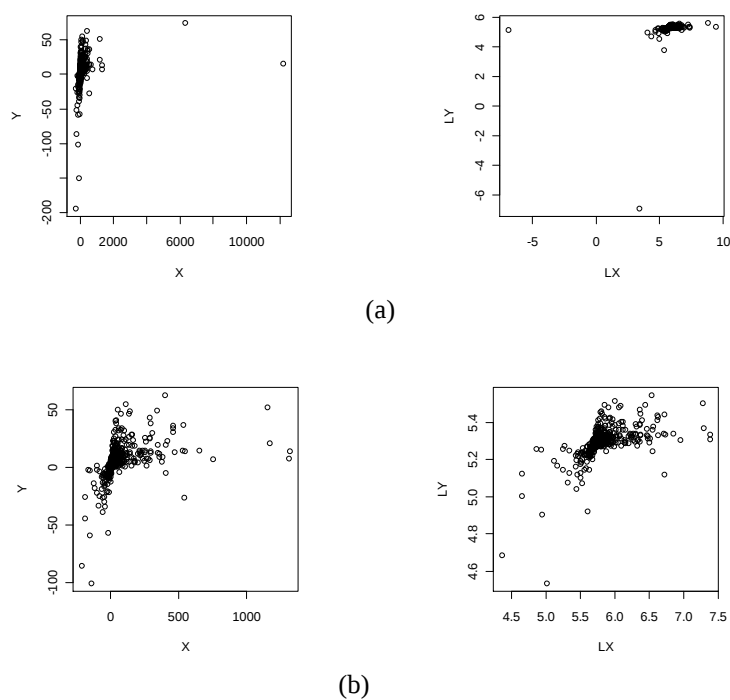
Figura 6 – Considerando o lucro líquido (X, em US$ milhões) e a margem sobre as vendas (Y, em %), temos os gráficos dos postos normalizados dos dados com outliers em (a) e sem 6 outliers em (b).
