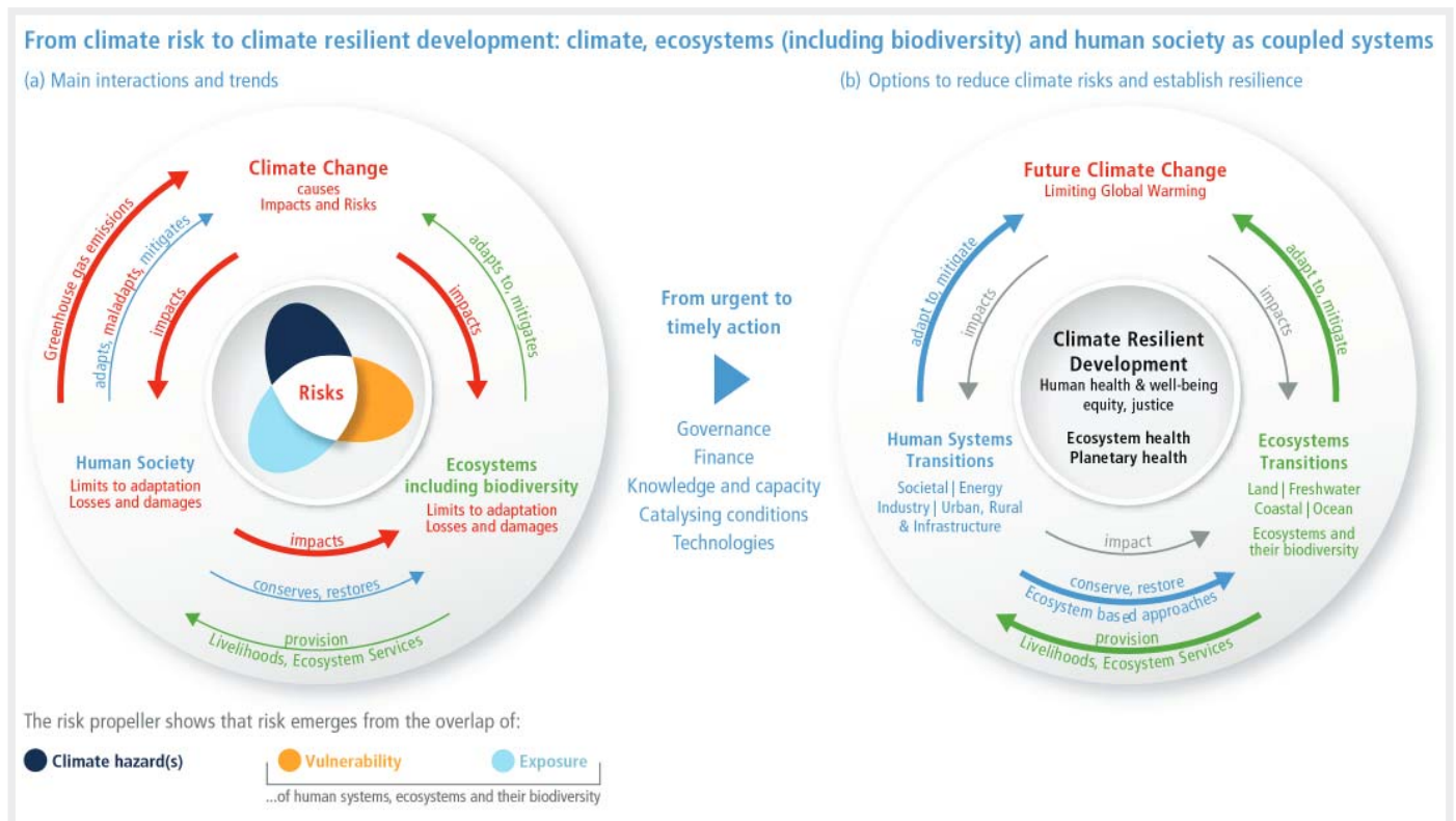
Figura 2. Ilustração das associações entre as mudanças climáticas, os sistemas humanos e os serviços ecossistêmicos, e de como poderemos construir um futuro mais resiliente, sustentável e justo, preservando os serviços ecossistêmicos através de estratégias de adaptação e mitigação. Fonte: IPCC WG2 SPM (Intergovernmental Panel on Climate Change, 2022) (Reprodução de figura e legenda autorizada). Crédito: "Figure SPM.1" (Intergovernmental Panel on Climate Change, 2022, p. 8).
