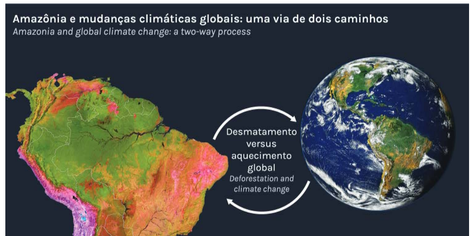
Figura 3. Interações entre as emissões do desmatamento e seus impactos no aquecimento global, e como o aquecimento global impacta no ecossistema amazônico.
