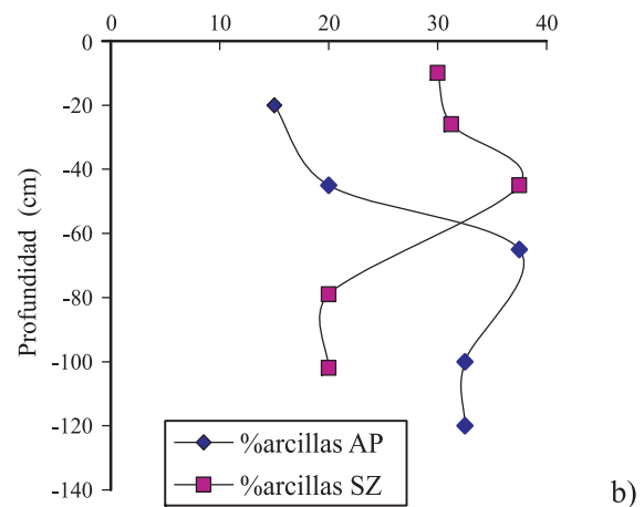
Figura 2. Variación del contenido de arcillas (%) con la profundidad en los suelos estudiados. R1, R2 y R3: Verónica; AP y SZ: Zárate, Argentina.
