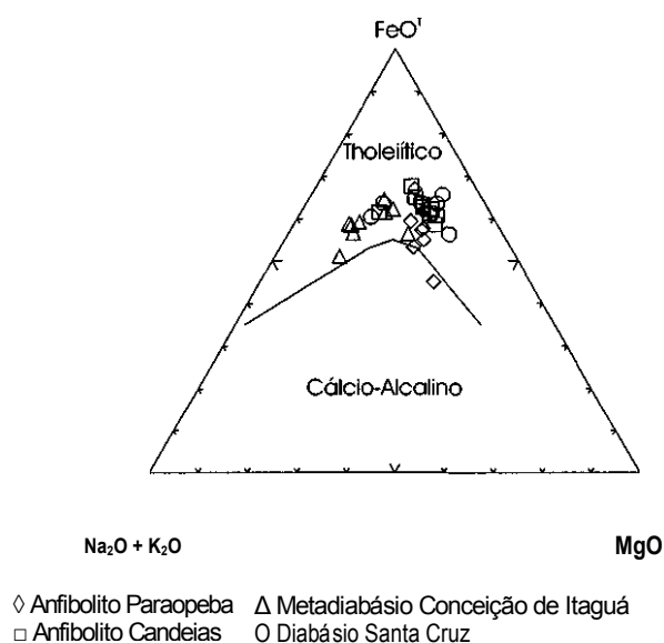
Figura 4 - Classificação geral das quatro gerações de diques máficos do Complexo Metamórfico Bonfim Setentrional de acordo com o diagrama AFM, segundo a proposta de Irvine & Baragar (1971).
