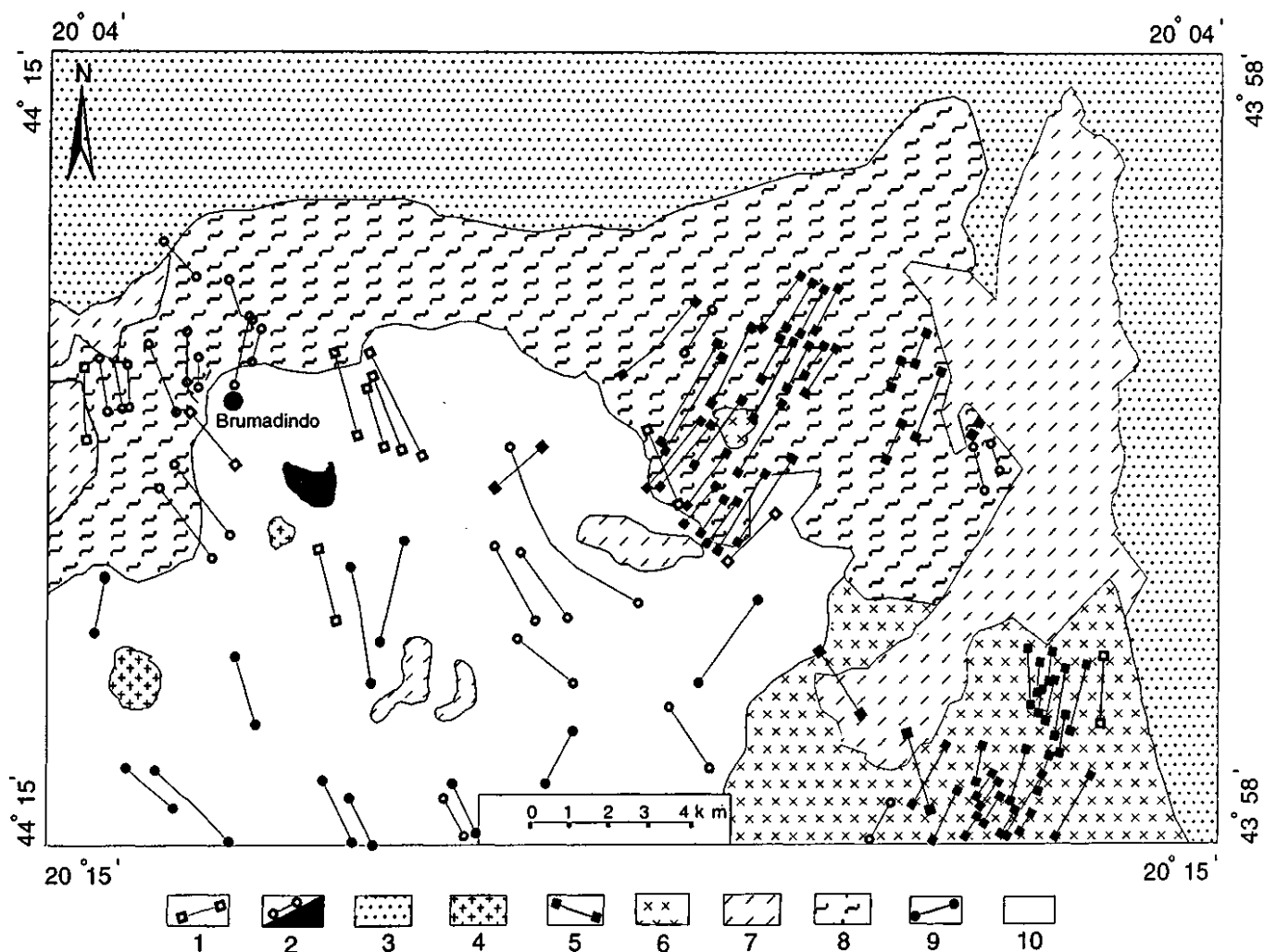
Figura 2 - Mapa geológico do Complexo Metamórfico Bonfim e de parte das sequências supracrustais do Quadrilátero Ferrífero (modificado de Carneiro et al 1997). Símbolos: 1 - Diabásio Santa Cruz; 2 - Metadiabásio Conceição do Itaguá; 3 - Super grupo Minas; 4 - Granito Brumadinho; 5 - Anfíbolito Candeias; 6 - Tonalito Samambaia; 7 - Supergrupo Rio das Velhas; 8 - Gnaiss Souza Noschese; 9 - Anfíbolito Paraopeba; 10 - Gnaiss Alberto Flores.
