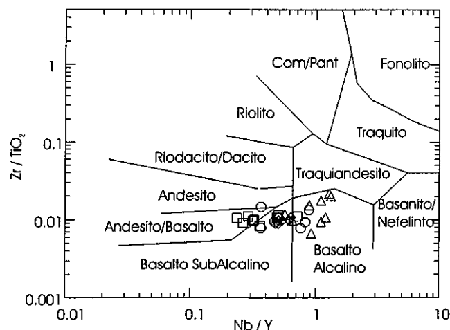
◇ Anfíbolito Paraopeba △ Metadiabásio Conceição de Itagua □ Anfíbolito Candeias ○ Diabásio Santa Cruz
