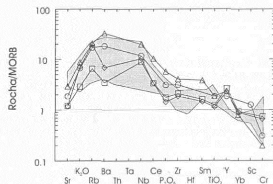
◇ Anfibolito Paraopeba △ Metadiabásio Conceição de Itaguá □ Anfibolito Candeias ○ Diabásio Santa Cruz
