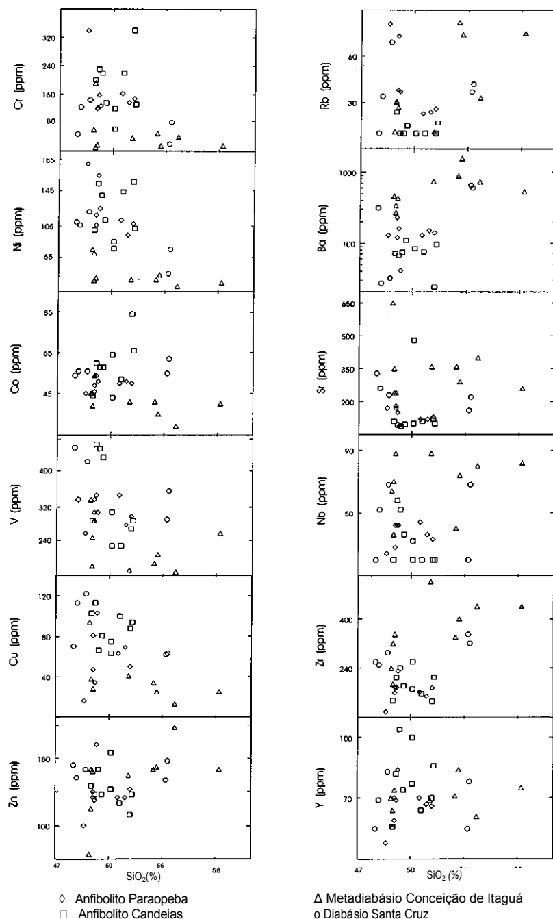
Figura 7 - Diagramas de variação ( \text{SiO}_2 versus Elementos Traços) para as quatro gerações de diques máficos do Complexo Metamórfico Bonfim Setentrional.
