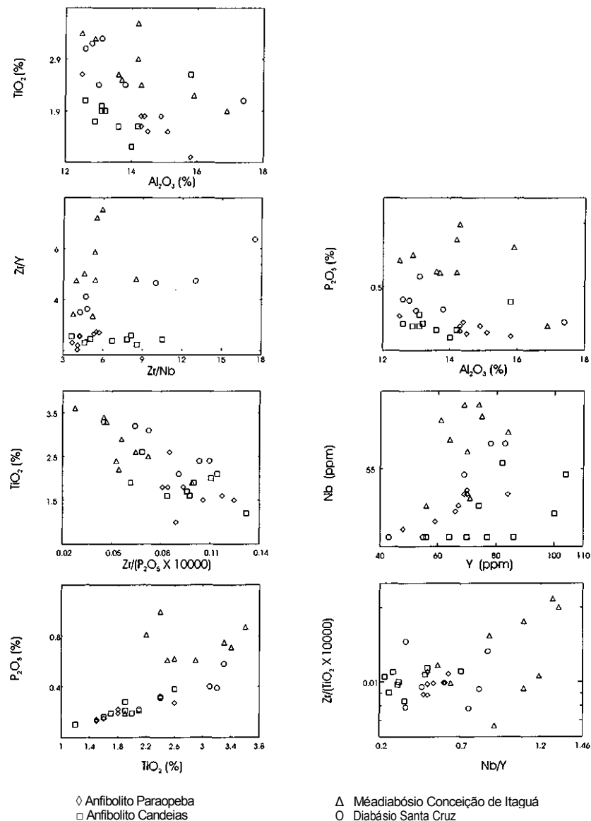
Figura 8 - Diagramas de variação para alguns elementos e/ou razões de elementos de potencial iônico intermediário das quatro gerações de diques máficos do Complexo Metamórfico Bonfim Setentrional.
