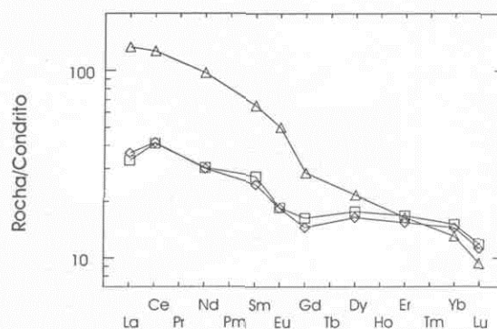
◇ Anfibolito Paraopeba △ Metadiabásio Conceição de Itaguá □ Anfibolito Candeias
