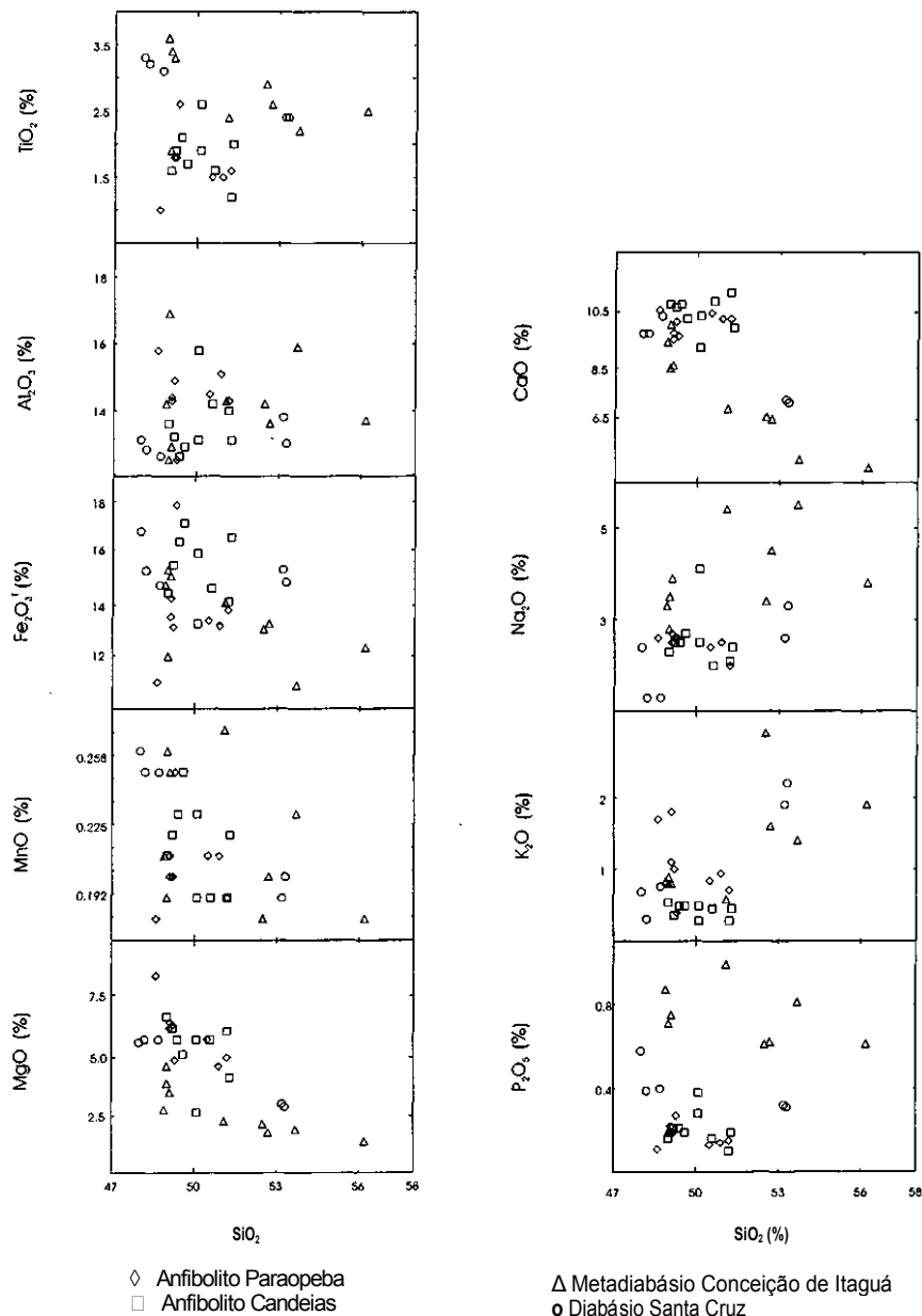
Figura 6 - Diagramas de variação ( \text{SiO}_2 versus Óxidos) para as quatro gerações de diques máficos do Complexo Metamórfico Bonfim Setentrional.
