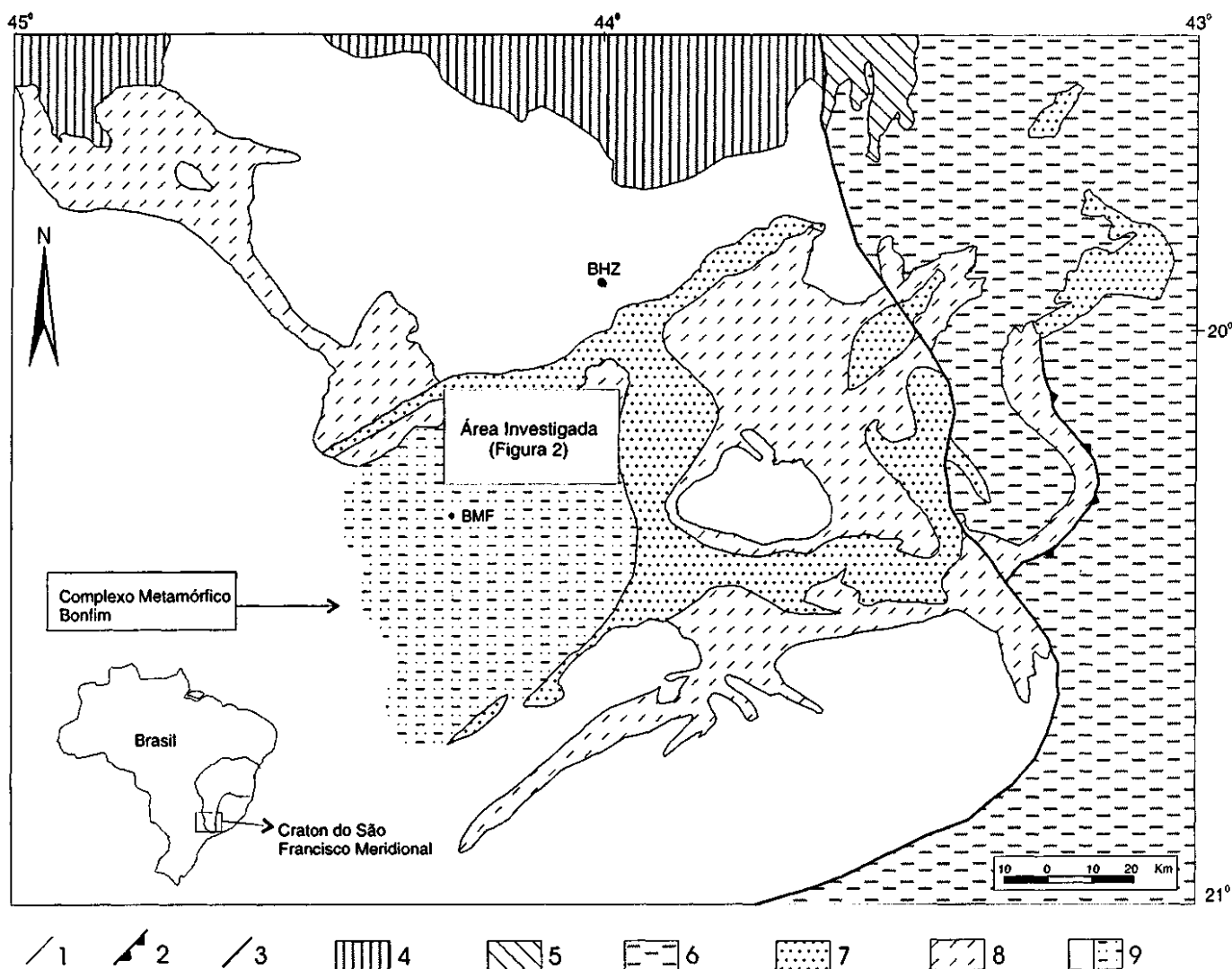
Figura 1 - Geologia do Craton do São Francisco Meridional (modificado de Carneiro 1992, Carneiro et al. 1997). Símbolos: 1 - Contato geológico; 2 - Empurrão; 3 - Limite cratônico oriental; 4 - Supergupo São Francisco; 5 - Supergupo Espinhaço; 6 - Complexo Metamórfico formado ou retrabalhado no Neoproterozóico; 7 - Supergupo Minas; 8 - Supergupo Rio das Velhas; 9 - Complexo Metamórfico Arqueano. BHZ - Belo Horizonte; BFM - Bonfim.
