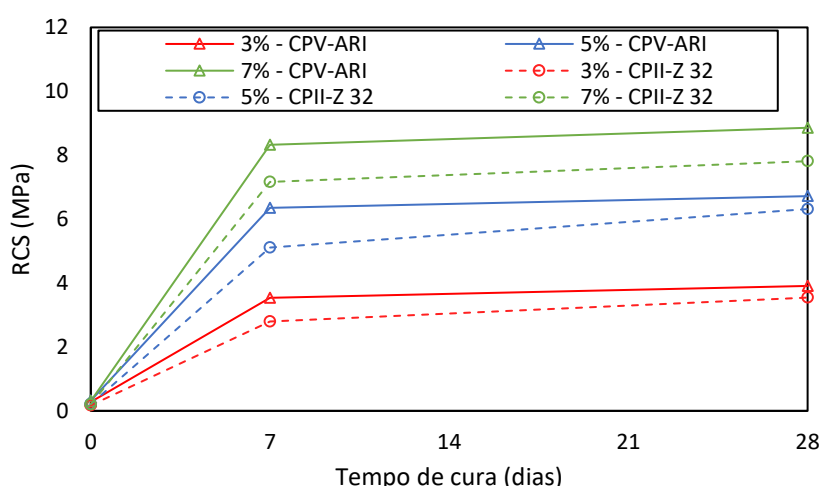
Figura 4: RCS das misturas SAC ao longo do tempo de cura.
