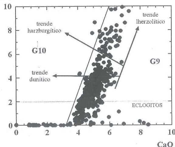
Figura 1: Diagrama CaO - Cr_2O_3 (Gurney 1985) mostrando que a maior parte das granadas estudadas são de natureza lherzolítica, seguidas por eclogíticas, além de harzburgíticas e duniticas, havendo também uma população derivada de rochas do embasamento.
