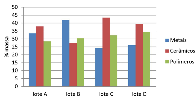
Figura 10. Gráfico de % massa de cada fração nos lotes.
