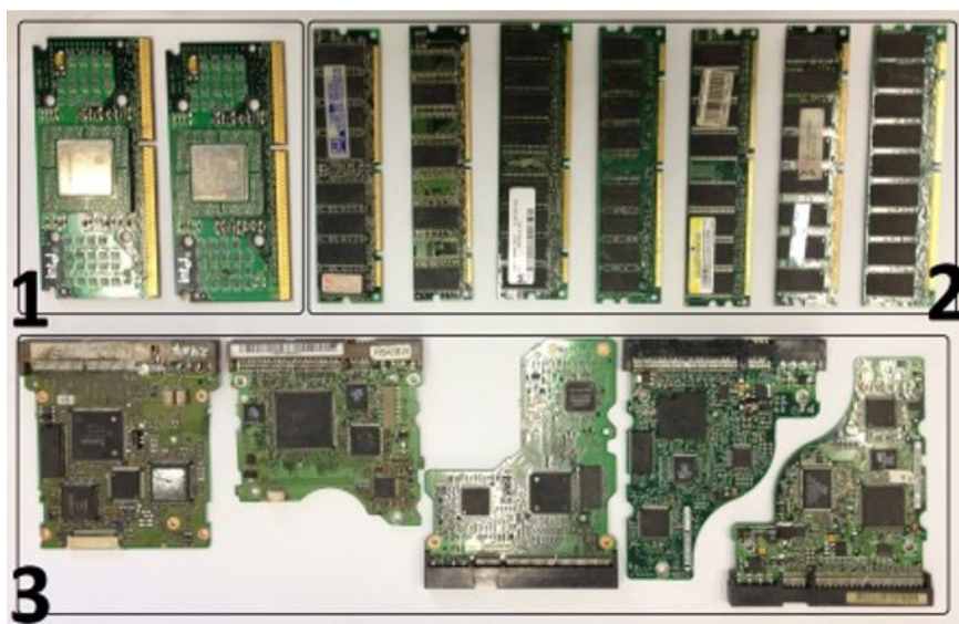
Figura 1. Lote A. 1-Memória dourada; 2-Procesador slot; 3-Placas de HD.
