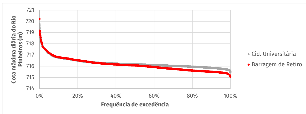
Figura 3: Curva de permanência do nível d'água máximo diário do Rio Pinheiros, para dois postos próximos da área de estudo (SAISP, 2022)
