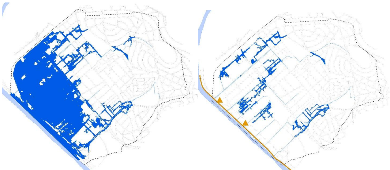
Figura 4: Manchas simuladas para condição de Tr 5 anos e nível do Rio Pinheiros em 720,21 m: cenário hidráulico atual (esquerda); cenário com as obras dos pôlderes, dique e válvula unidirecional (direita)
