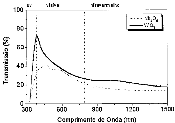
Figura 4: Comparação entre as curvas de transmissão espectral do vidro eletocrômico com filme de WO_3 e do vidro eletocrômico com filme de Nb_2O_5 no estado polarizado.
