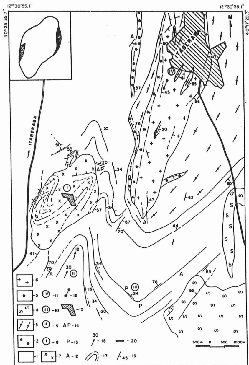
Fig. 1 - Mapa geológico da Região de Itaberaba, com as ocorrências de molibdenita. 1 - gnaisses granitoides; 2 - gnaisses bandados; 3 - gnaisses kinzigíticos; 4 - gnaisses hornblenda-biotita migmatíticos com intercalações anfibolíticas (Domínio Migmatítico); 5 - Maciço de Itaberaba; 6 - fácies fino a biotita + granada; 7 - fácies porfiróide a biotita; 8 - Maciço de Pedra d'Água; 9 - hipersthênio-(granada) granitos e aplo-pegmatitos. Ocorrências de Molibdenita: 10 - Fazenda Pedra d'Água; 11 - Fazenda Pedra d'Água Sul; 12 - Fazenda Lajedinho; 13 - Rio Piranhas; 14 - corpo aplítico; 15 - corpo pegmatítico; 16 - corpo aplo-pegmatítico; 17 - área mineralizada da Fazenda Pedra d'Água; 18 - dique aplo-pegmatítico; 19 - planos de foliação; 20 - lineação; 21 - atitude de foliação; 22 - estrada.
