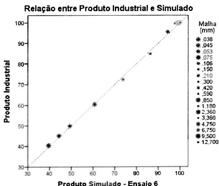
Figura 2. Gráfico produto industrial versus produto simulado – ensaio 6.
