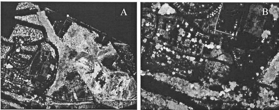
Figura 5-a) Composição colorida R:Clorofila total; G: Clorofila-a; B: Clorofila-b
