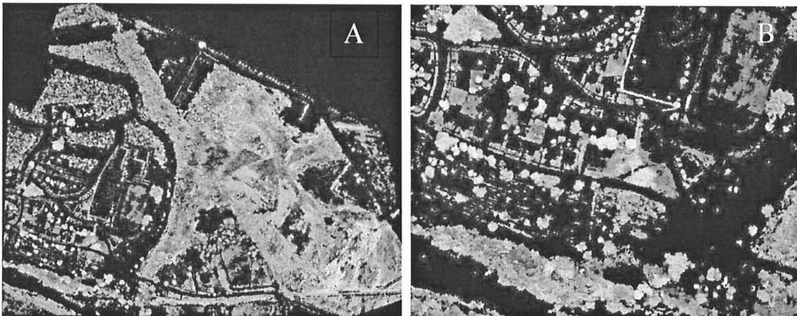
Figura 4-a) Composição colorida R:Carotenos; G:Água foliar; B:Clorofila total
