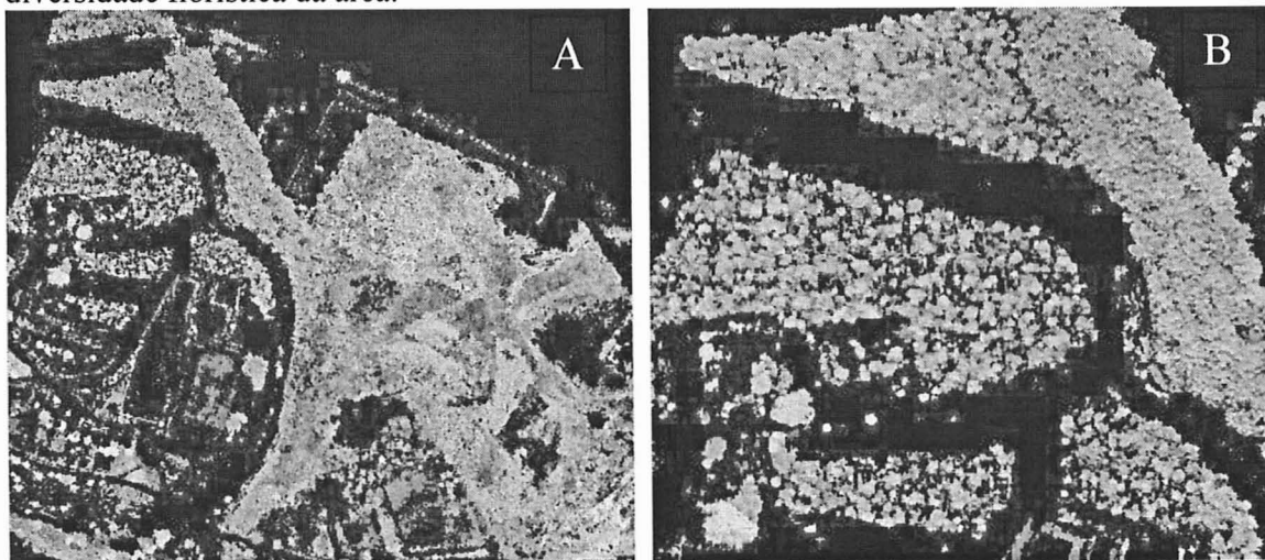
Figura 3-a) Composição colorida R:Antocianina; G:Água foliar; B:Carotenos 3-b) Ampliação da área com vegetação em diferentes estágios de regeneração e bambú.
