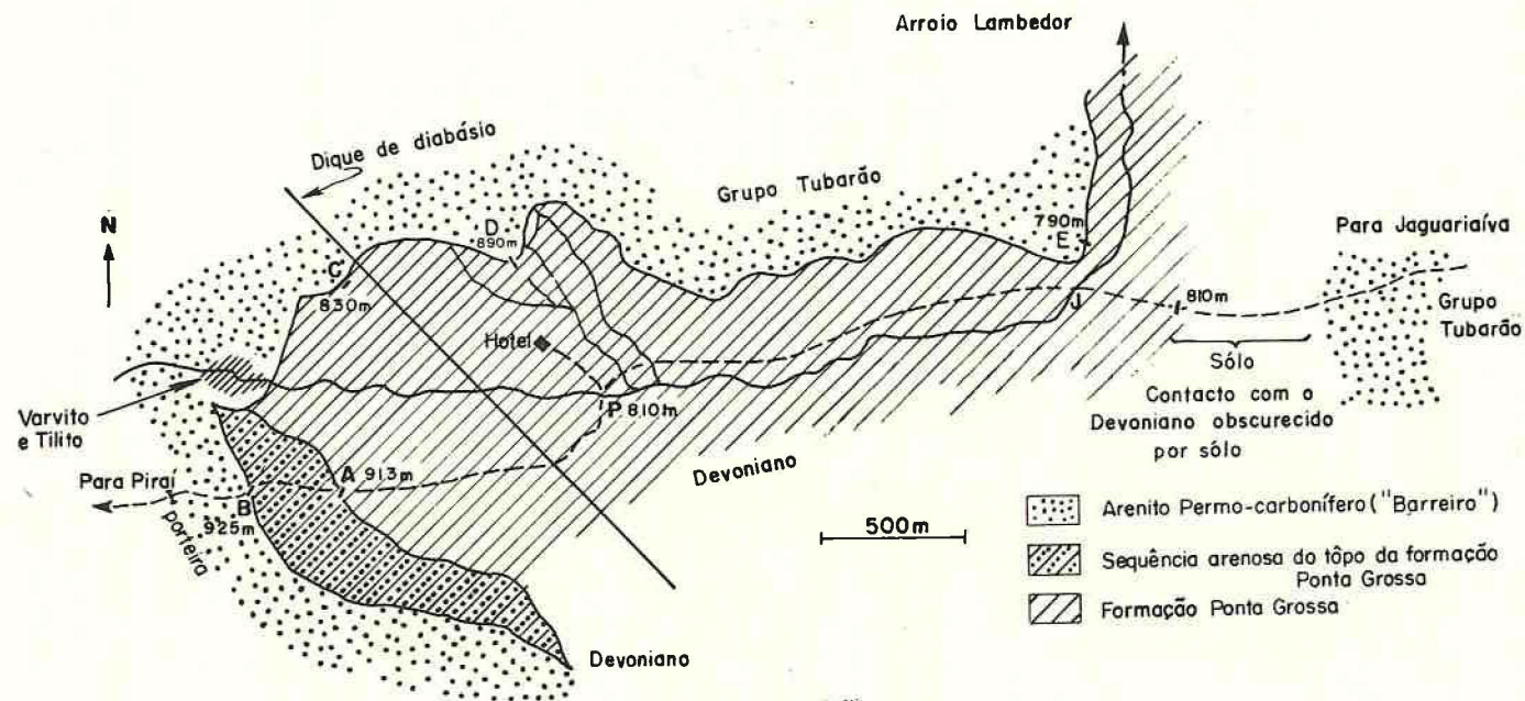
Fig. 2 — Esbôço geológico da região de Lamberdor, Paraná (Modificado de Petri, 1948).
