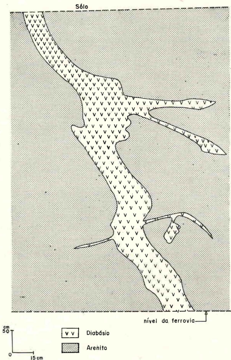
Fig. 5 — Pormenor do contato entre Arenito Furnas e diabásio. Corte da estrada de ferro Jaguariaíva-Arapoti, cêrca de 300 m adiante do km 7.
