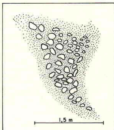
Fig. 1 — Conglomerado preenchendo calha formada por erosão fluvial. Arenito do Grupo Tubarão, Lamedor, Paraná.
