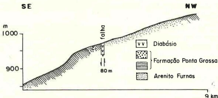
Fig. 4 — Perfil geológico retificado ao longo da estrada de ferro Jaguariaíva-Arapoti, entre os kms 2 e 14 (Modificado de Petri, 1948).
