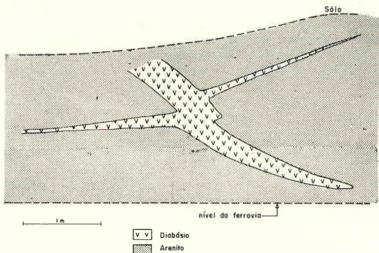
Fig. 7 — Pormenor do contato entre o Arenito Furnas e diabásio; mesma localidade da Fig. 5.
