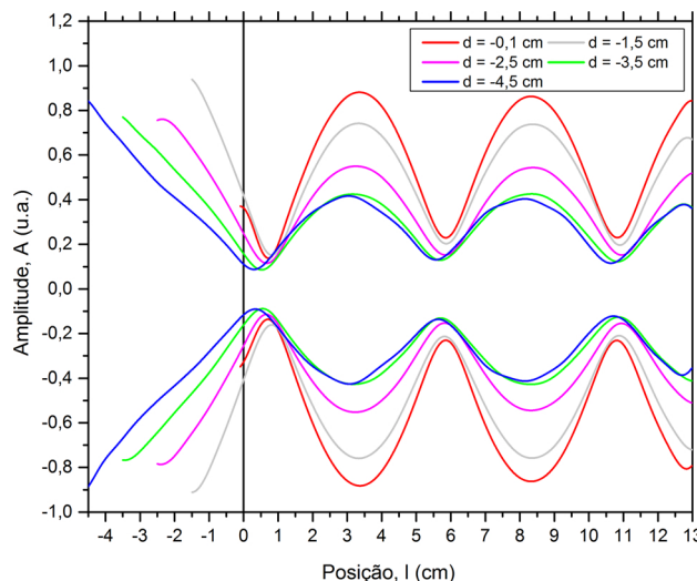
Figura 14: Envelope do sinal adquirido para uma frequência fixa, f_e = 3300 Hz, em um tubo aberto em uma extremidade (esquerda) e com comprimento fixo, L = 13,0 cm ( n = 3 , m = 2 ), não levando em consideração a aproximação terminal. As distâncias negativas representam a distância do alto-falante em relação à extremidade do tubo (posição l = 0,0 cm). Todas as medidas foram realizadas com a mesma amplitude na onda sonora aplicada. O microfone iniciou suas medidas da superfície do alto-falante, externo ao tubo.
