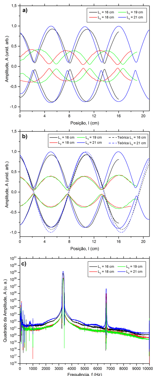
Figura 13: Sinais adquiridos para uma frequência de excitação de f_e = 3300 Hz e comprimentos L do tubo diferentes. a) Envelope dos sinais originais para cada comprimento L , sendo L = 21 cm o comprimento correspondente a n = m = 4 . b) Sinais espelhados na abcissa, e deslocados fazendo com que os finais das curvas do item a sejam coincidentes em l = 0,0 cm e comparados às curvas teóricas (tracejadas). A curva teórica para L = 21 cm foi determinada utilizando a frequência de excitação utilizada no experimento enquanto a curva teórica para L = 16 cm, que não corresponde exatamente a um comprimento cujo n resultante seria um inteiro foi simulada utilizando f = 3150 Hz para ilustrar o efeito de uma excitação não ideal. c) Transformada de Fourier do sinal original, evidenciando que a frequência característica é praticamente a mesma para todas as curvas adquiridas.
