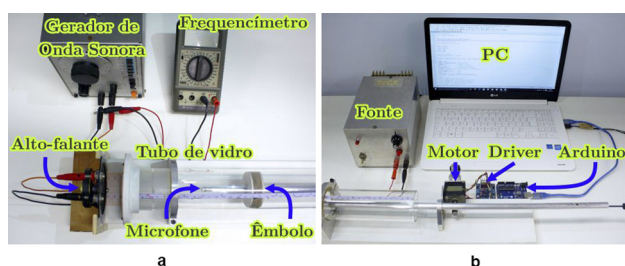
Figura 6: Foto da montagem experimental utilizada para aquisição de dados. a) Gerador de sinal e frequencímetro ligado ao alto falante, evidenciando também o tubo que contém o êmbolo e o microfone para aquisição com movimentação separada. b) Extremidade oposta do tubo onde o motor de passo faz o movimento do êmbolo ou microfone. O motor está ligado ao driver alimentado pela fonte e também ao Arduino controlado pelo computador.
