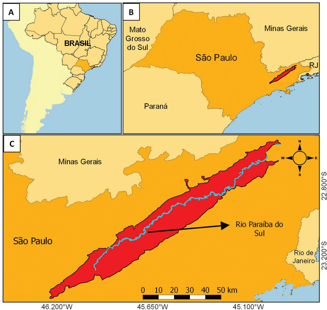
Figura 1. Mapa de localização da Bacia de Taubaté. A) Localização no Brasil; B) Localização no Estado de São Paulo; C) Delimitação da Bacia de Taubaté (em vermelho) com indicação do Rio Paraíba do Sul. Figure 1. Location map of the Taubaté Basin. A) Location in Brazil; B) Location in São Paulo State; C) Delimitation of Taubaté Basin (in red) indicating of the Paraíba do Sul River.
