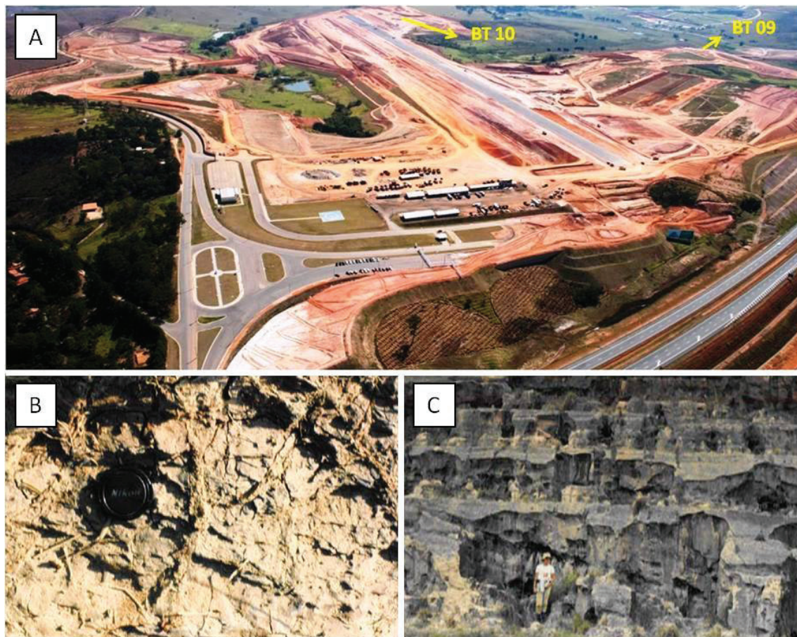
Figura 10. Exemplos de geossítios e potenciais geossítios que estão na iminência de desaparecer ou que já não existem mais. A) Obras da construção do aeroporto de Caçapava – SP, o Aerovale, com indicação de dois geossítios (BT-09 e BT-10, em amarelo). Fonte: www.aerovale-cea.com.br/empreendimento (Acesso em: 11 ago. 2017); B) Afloramento com gretas de contração que foi destruído para construção de via de acesso para a cidade de Campos do Jordão – SP; C) Afloramento com arenitos estratificados que foi destruído para construção de estrada secundária na região de Tremembé – SP. Figuras B e C extraídas de Riccomini (1989).
