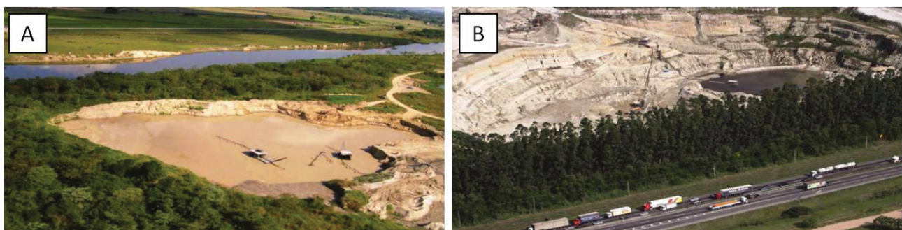
Figura 9. Áreas de mineração de areia na região da Bacia de Taubaté. A) Cava de extração de areia invadindo área de preservação e destruindo mata ciliar próximo ao Rio Paraíba do Sul; B) Desmonte hidráulico em Jacareí, às margens da Rod. Dutra. Notar a barreira de eucaliptos plantada ao longo da rodovia para ocultar as cavas. Fonte: http://www.quimicosjc.org.br/pdfs/especiais/Cavas-de-areia-2012.pdf (Acesso em: 02 set. 2017).
