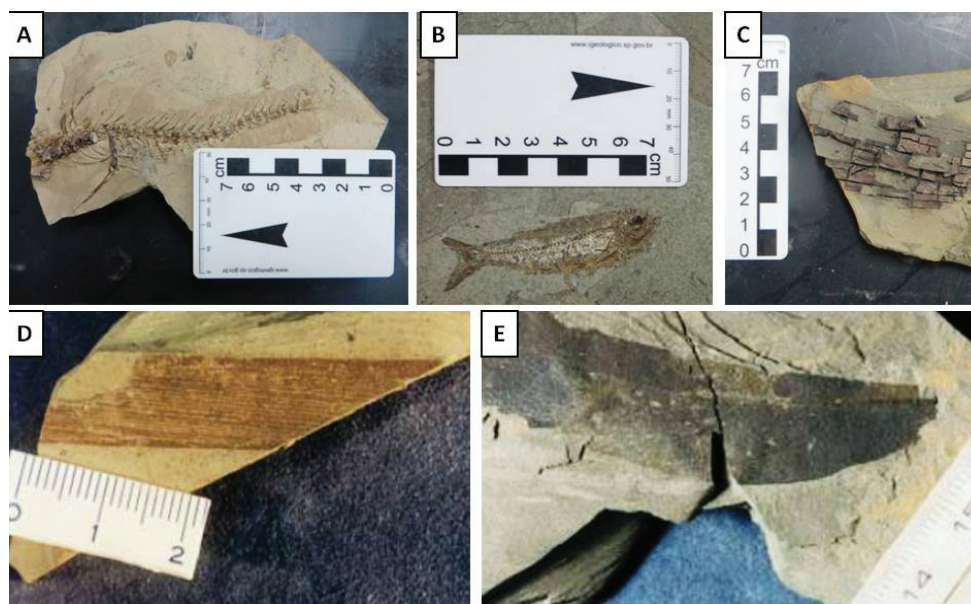
Figura 5. Geossítios paleontológicos da categoria geológica "Abertura da bacia". A) Fóssil de espinho de peixe; B) Fóssil de peixe completo; C) Fóssil de parte de tronco de árvore. Coletados pelo Prof. Luiz Eduardo Anelli durante trabalhos de campo na área do geossítio (Fonte: Coleção didática do IGC/USP); D) Tronco fóssil (Família Typhaceae-Typha tremembensis); E) Folha fóssil (Família Sapindaceae). Coletados no "Jazigo Quiririm". Imagens: Maria Judite Garcia.
