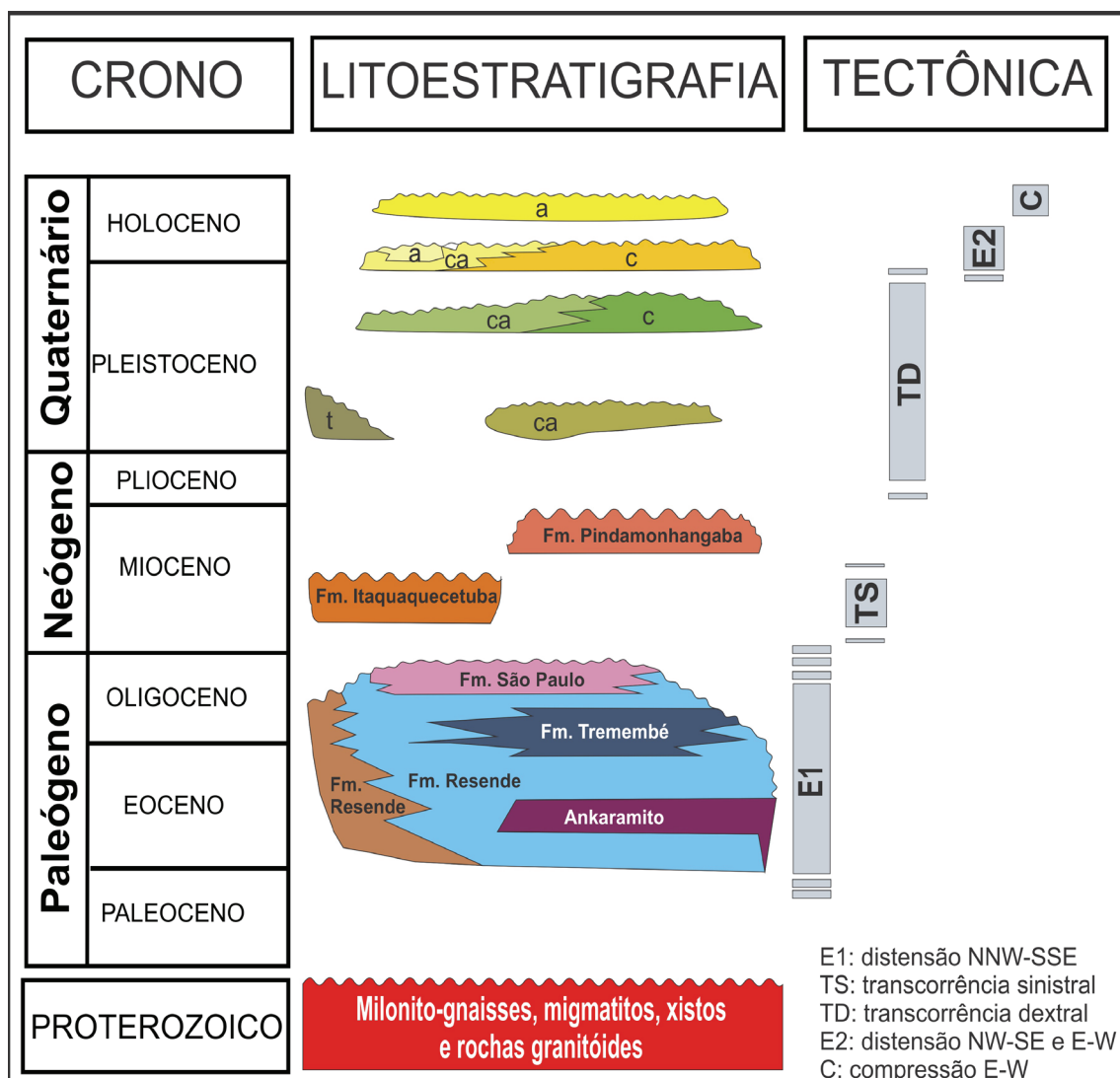
Figura 2. Litoestratigrafia e evolução tectono-sedimentar do segmento central do Rifte Continental do Sudeste do Brasil (Riccomini, 1989).
