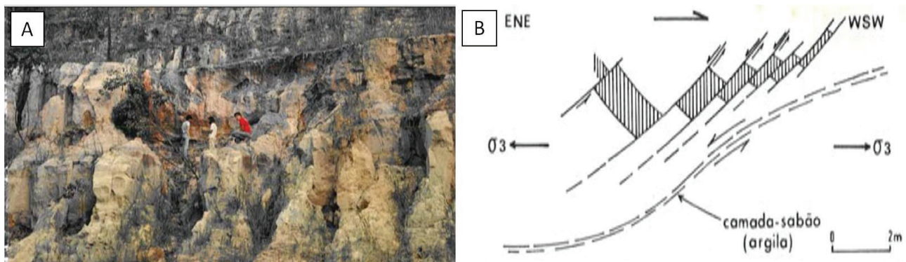
Figura 8. Geossítio Falhas conjugadas da Formação Pindamonhangaba. A) Vista geral do afloramento na década de 1980 (Fonte: Riccomini, 1989); B) Esquema do afloramento indicando falhas em arranjo dominó e camada-sabão em grande escala, não mais visíveis (Riccomini, 1989).
