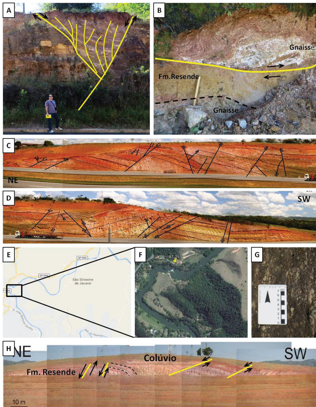
Figura 6. Geossítios da categoria geológica "Deposição e deformação neógena". A) Conjunto de falhas normais, pós-sedimentares, com mergulhos moderados a altos, direção NNE-SSW. Algumas das falhas provavelmente resultam da reativação de falhas transcorrentes mais antigas e apresentam estrutura em flor negativa; B) Contato tectônico entre o gnaissse do embasamento e os diamictitos da Formação Resende (em amarelo). Em preto pontilhado, contato erosivo; C) Lado esquerdo do afloramento, com indicação das falhas normais afetando as rochas da Formação Resende e colúvios quaternários; D) Lado direito do afloramento, com indicação das demais falhas (Moura, 2015); E) Localização do geossítio com indicação do cotovelo de captura. Fonte: Google Earth; F) Vista de cima do afloramento. Fonte: Google Earth; G) Detalhe do gnaissse pré-cambriano orientado para NE com cristais de feldspato bem desenvolvidos; H) Falhas rotacionais de baixo mergulho. Imagens: Daniel do Valle.
