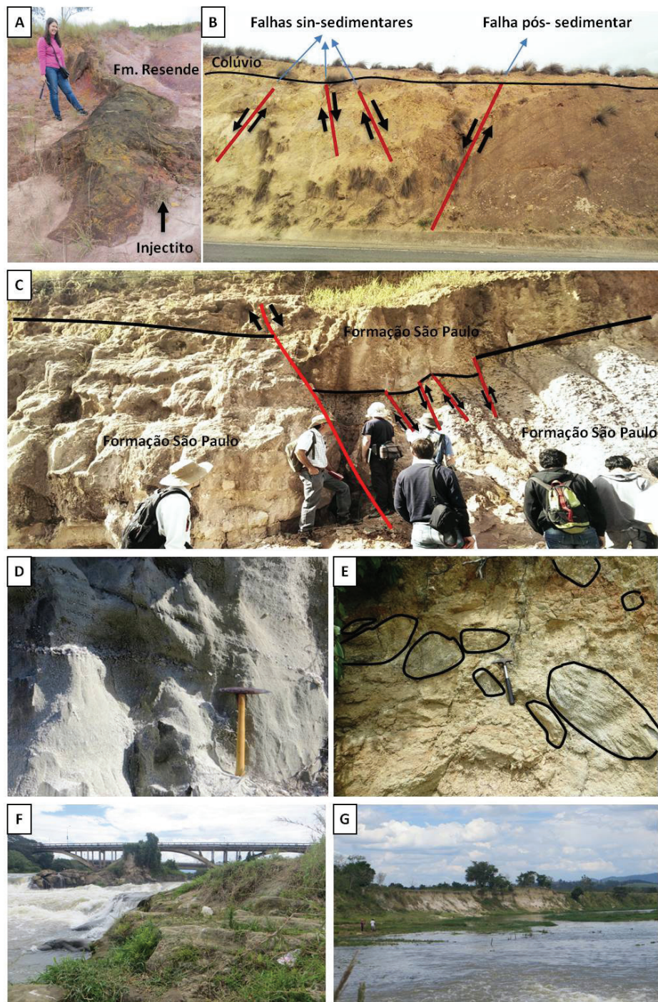
Figura 4. Geossítios da categoria geológica “Abertura da bacia”. A) Dique de material arenoso cortando argilitos da Formação Resende; B) Falhas sin-sedimentares que afetam os argilitos da Formação Resende. Observar, no lado direito da fotografia, a falha principal de direção NE-SW, que marca o contato entre embasamento pré-cambriano e a Formação Resende; C) Falha normal de direção NE-SW que deforma as rochas da Formação São Paulo e falhas inversas no lado direito da imagem; D) Lentes com conglomerado clasto suportado na base em contato com arenito mais fino na base, ilustrando a deposição intercalada de grãos mais grossos e finos; E) Depósito de leque aluvial com a presença de blocos decimétricos do embasamento; F) Embasamento granítico pré-cambriano, muito alterado, que aflora no leito do Rio Paraíba do Sul; G) Sedimentos quaternários depositados na borda do rio.
