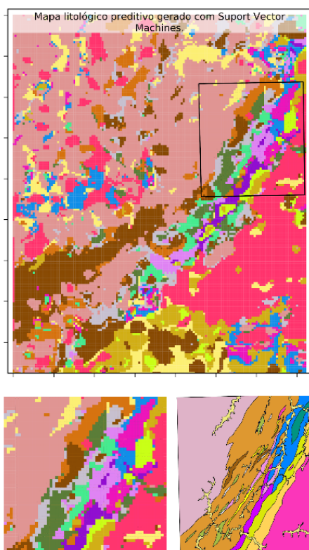
Figura 1: Resultados da classificação por SVM.
