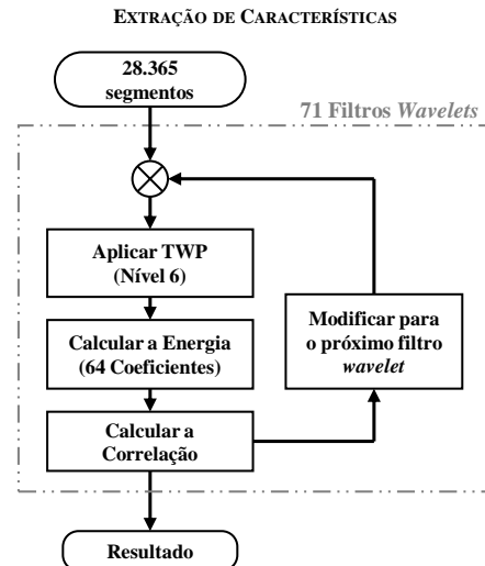
Fig. 2. Procedimento de extração de características dos segmentos.
