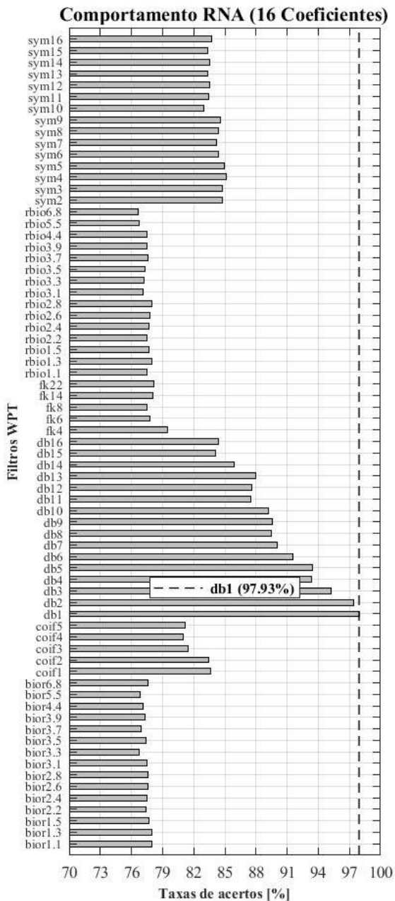
Fig. 7. Comportamento RNA com os 16 coeficientes mais correlacionados.
