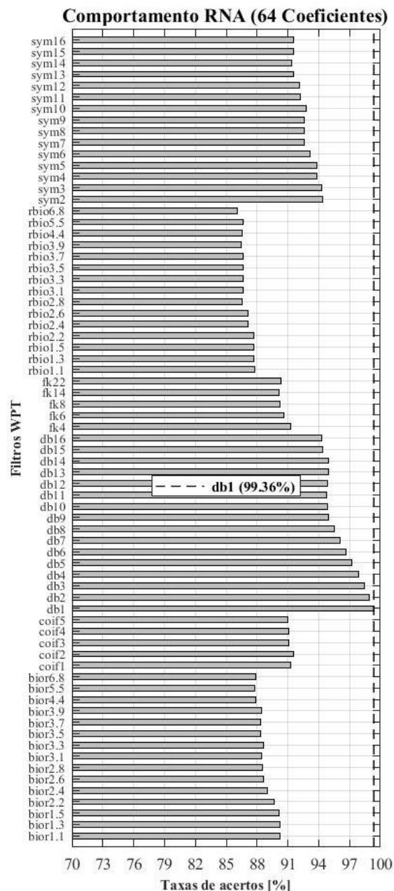
Fig. 10. Comportamento RNA com todos coeficientes.
