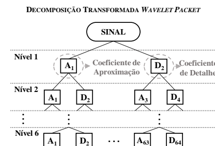
Fig. 3. Decomposição da TWP para o nível 6.
