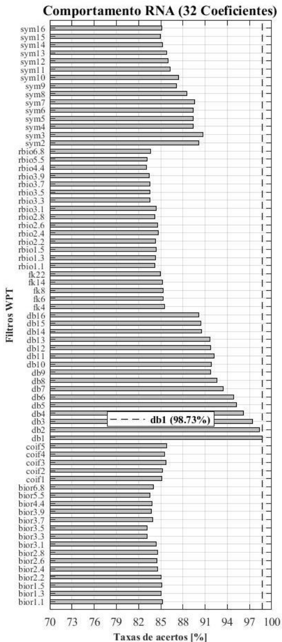
Fig. 9. Comportamento RNA com os 32 coeficientes mais correlacionados.
