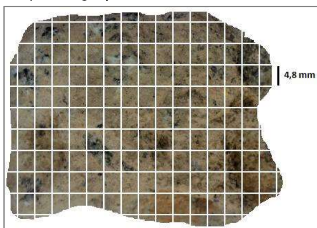
Figura 3 - Análise textural para configuração de britadores
