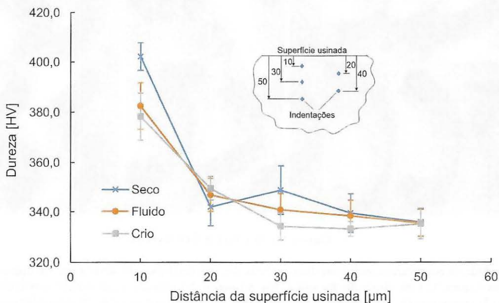
Figura 6. Perfil da microdureza ao longo da seção transversal da peça. Coeficiente de variação (CV): (a) 2,08% a seco, (b) 1,95% com fluido convencional e (c) 1,63% com fluido criogênico
