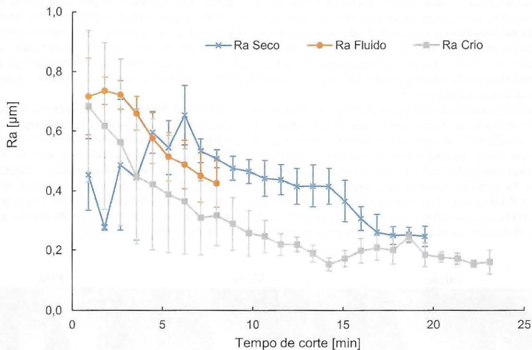
Figura 5. Desvio médio aritmético (Ra). Coeficientes de variação (CV): 16,3% a seco, 13,9% com fluido convencional e 27,2% com fluido criogênico.
