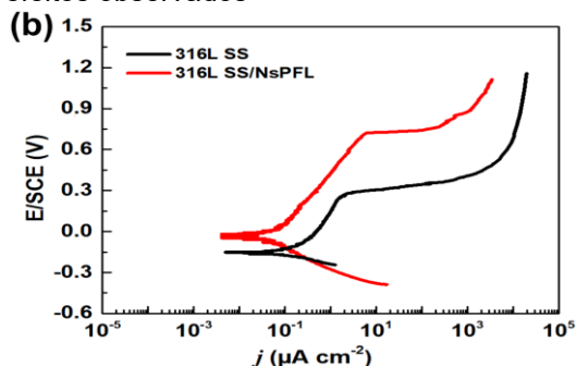
Figura 1. (a) Comparação das curvas de OCP e (b) comparação das curvas de polarização potenciodinâmica para o aço 316L com e sem tratamento à laser.
