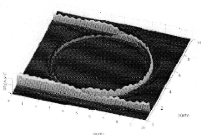
Fig. 6. Distribuição de intensidade de campo em um comprimento de onda fora da ressonância do filtro (ponto B das Figs. 3 e 4).
