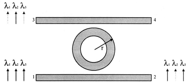
Fig. 1. Filtro óptico com anel como elemento ressonante onde o acoplamento com os guias é obtido por meio de campo evanescente. Apenas o comprimento de onda \lambda_2 (para o qual o anel foi projetado) acopla-se ao guia de saída via anel ressonante. Os outros comprimentos de onda não sofrem alteração de trajetória. A janela antes ocupada por \lambda_2 pode ser ocupada por outros sinais da rede pela inserção de novo comprimento de onda.
