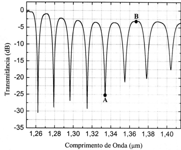
Fig. 3. Característica de transmitância na porta 2 do filtro ressonador em anel.
