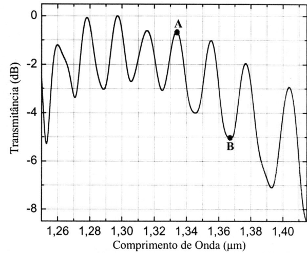
Fig. 4. Característica de transmitância na porta 3 do filtro ressonador em anel.
