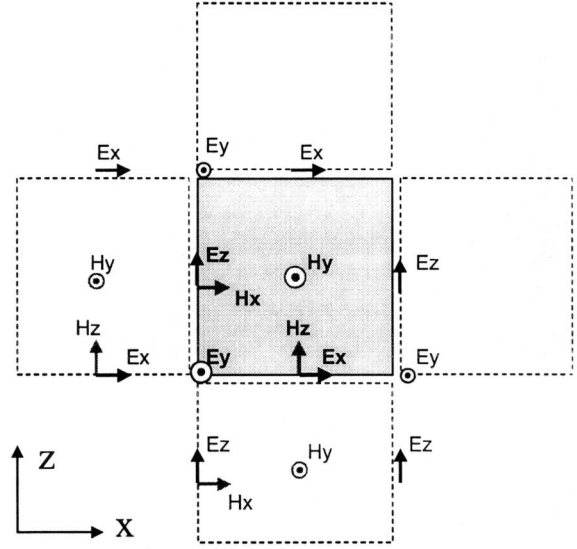
Fig. 2. Célula de Yee Bidimensional [13].
