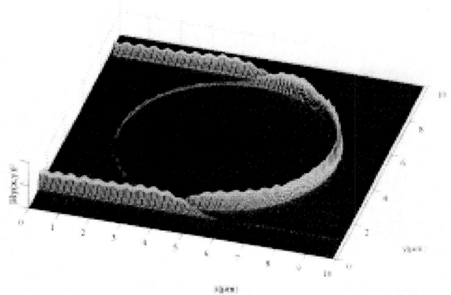
Fig. 5. Distribuição de intensidade de campo em um comprimento de onda de ressonância do filtro (ponto A das Figs. 3 e 4).
