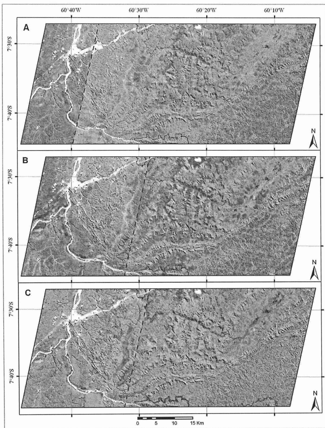
Figura 2. Composições coloridas RGB combinando PCs, derivadas das APCs sobre as razões de bandas, após filtragem passa-baixa e introdução de imagem de albedo. A. Resultado da APC baseada na matriz de correlação (16jul2000: PC1,-PC2,PC7; 4jul2007: PC1,-PC2, PC8). B, C. Resultados das APCs baseadas nas matrizes de covariância. B. (PC1a, PC3c, -PC1b). C. (PC3c, PC2c, -PC1b). Em tracejado o limite entre os mosaicos 16jul2000 e 4jul2007.
