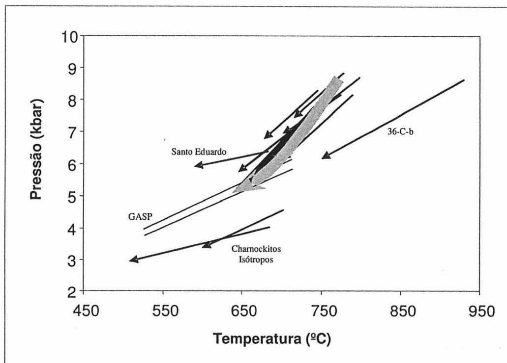
Figura 1 – Evolução P-T-t das rochas da região de São Fidelis (a seta a cinzento indica a tendência geral de arrefecimento e descompressão das rochas da região de São Fidelis). As litologias com um percurso P-T-t diverso estão individualizadas. GASP – equilíbrio 3 Anortite = Grossulária + 2 \text{Al}_2\text{SiO}_5 + \text{SiO}_2 (Newton & Haselton, 1981) referente aos bordos minerais da Unidade São Fidelis.
