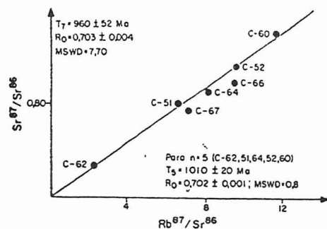
Fig. 4 - DIAGRAMA ISOCRÔNICO DE REFERÊNCIA PARA GNAISSES MICÁCEOS (UNIDADE VASSOURASI) E MIGMATITOS DO "COMPLEXO SALGUEIRO-CACHOEIRINHA" (de Brito Neves et al, 1984)
