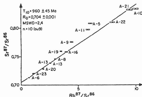
Fig. 5 - DIAGRAMA ISOCRÔNICO DE REFERÊNCIA PARA AS AMOSTRAS DA "SÉRIE DBSA" MIGMATITOS E GNAISSES DA UNIDADE A ("COMPLEXO CABROBÓ") AO NORTE DE CABROBÓ-PE. (de Brito Neves et al, 1984)
