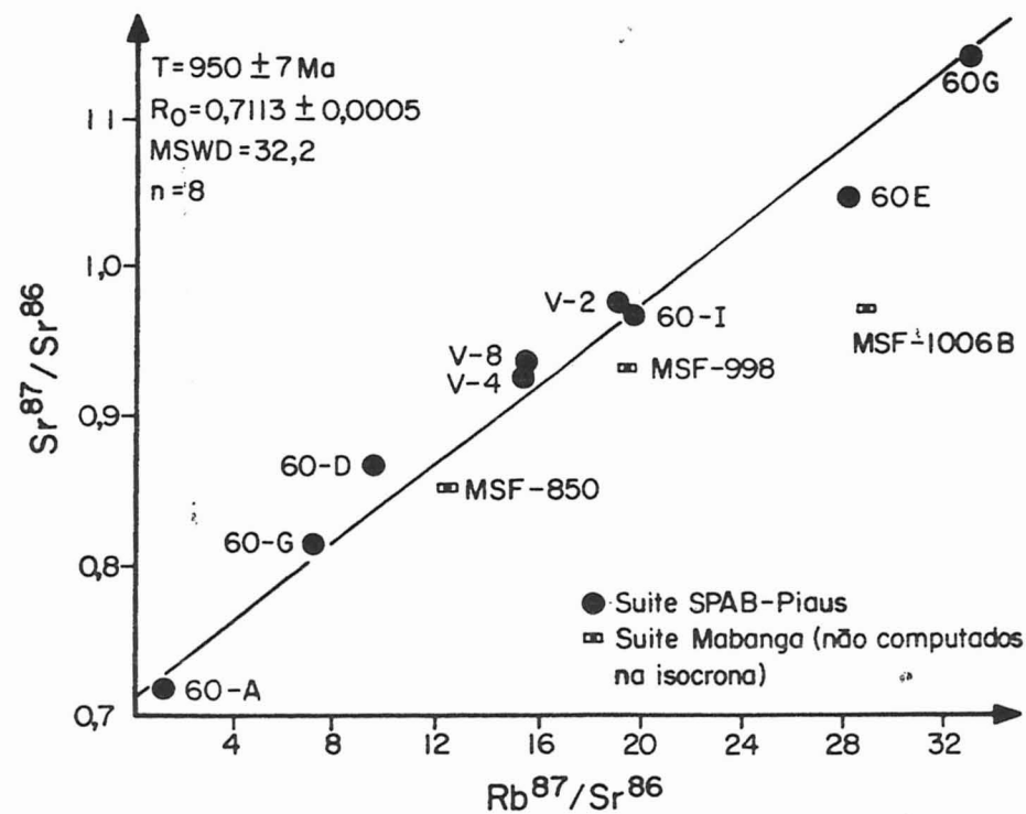
Fig. 3 - DIAGRAMA ISOCRÔNICO PARA AS META-VULCÂNICAS ÁCIDAS (ORTOGNAISSES) DE PIAUS, PA.
