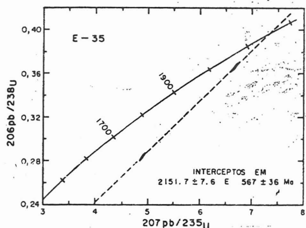
FIGURA 2 — DIAGRAMA CONCORDIA COM DADOS U-Pb PARA O EMBASAMENTO (LITOLOGIAS DO GRUPO SÃO VICENTE), (E-26 — BIOTITA — GRANODIORITO, E-26 — HORNBLENDA — BIOTITA — GNAISSE, E-35 — METAGABRO).
