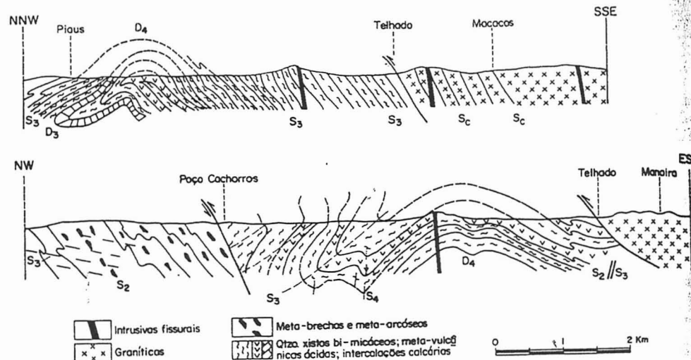
Fig. 1- SECCOES GEOLÓGICAS ESQUEMÁTICAS TRANSVERSAIS DA ÁREA DE COLETAS EM PIAUS E NORTE DE MANAIRA-PB
