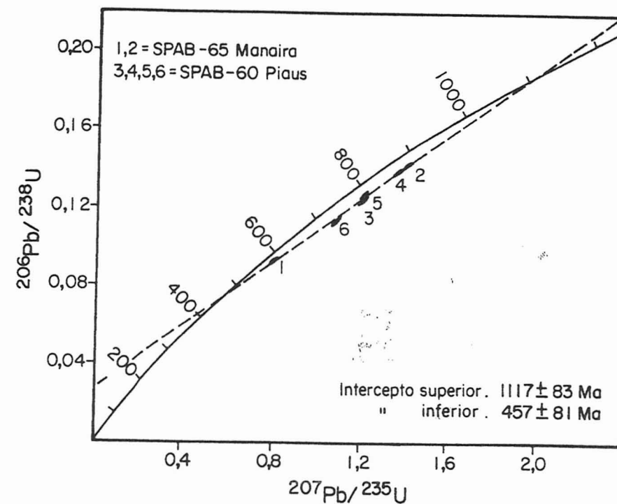
Fig. 2- DIAGRAMA DISCÓRDIA PARA ZIRCÕES DAS META-VULCÂNICAS DO NORTE DE MANAIRA (SPAB-65) E PIAUS (SPAB-60)-PA.
