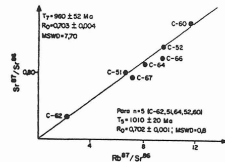
Fig. 4 - DIAGRAMA ISOCRÔNICO DE REFERÊNCIA PARA GNAISSES MICÁCEOS (UNIDADE VASSOURA) E MIGMATITOS DO "COMPLEXO SALGUEIRO-CACHOEIRINHA" (de Brito Neves et al, 1984)
