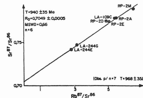
Fig. 6 - DIAGRAMA ISOCRÔNICO PARA O AUGEN-GNAISSE (SIN-TANGENCIAL, D2) NAS IMEDIAÇÕES DE AFRÂNIO-PE (SISTEMA RIACHO DO PONTAL). (mod. de Jardim de Sá et al, 1988)
