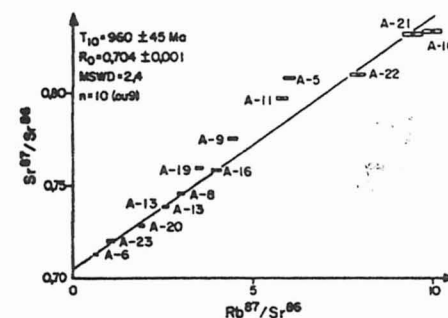
Fig. 5 - DIAGRAMA ISOCRÔNICO DE REFERÊNCIA PARA AS AMOSTRAS DA "SERIE DBSA" MIGMATITOS E GNAISSES DA UNIDADE A ("COMPLEXO CABROBÓ") AO NORTE DE CABROBÓ-PE. (de Brito Neves et al, 1984)
