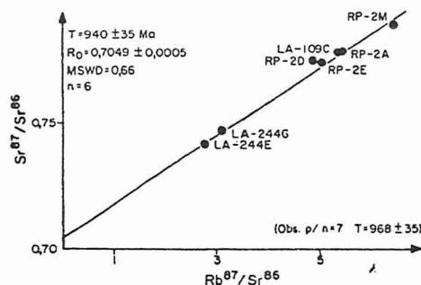
Fig. 6 - DIAGRAMA ISOCRÔNICO PARA O AUGEN-GNAISSES (SIN-TANGENCIAL, D2) NAS IMEDIAÇÕES DE AFRÂNIO-PE (SISTEMA RIACHO DO PONTAL). (mod. de Jardim de Sá et al, 1988)
