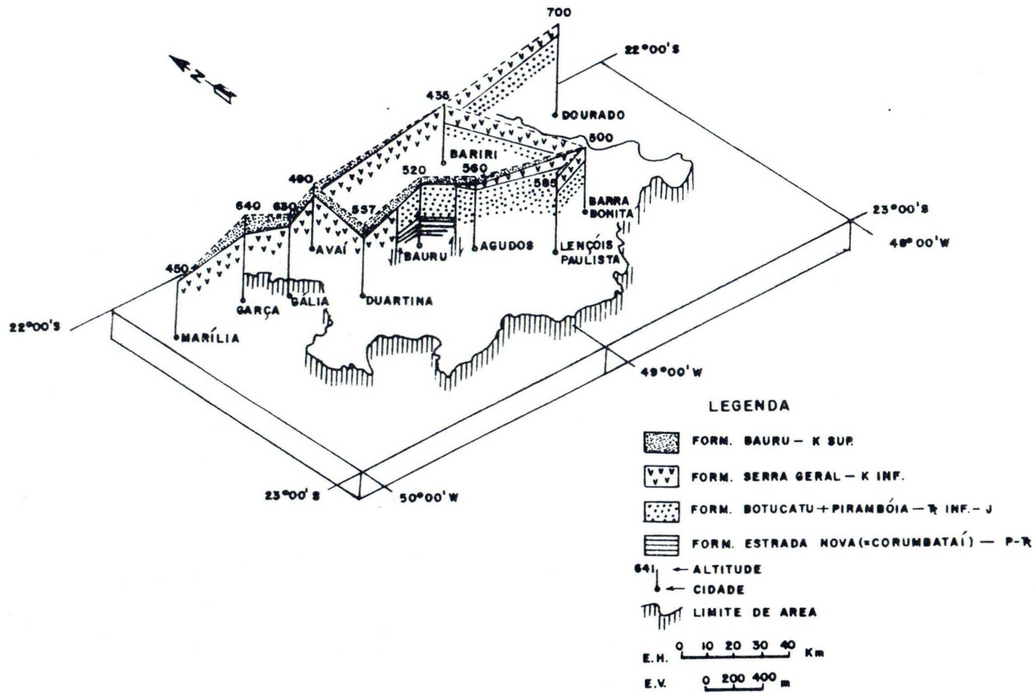
FIG. 3 — DIAGRAMA EM PAINEL DA FORMAÇÃO BAURU NA REGIÃO DO "HORST" DE BAURU
