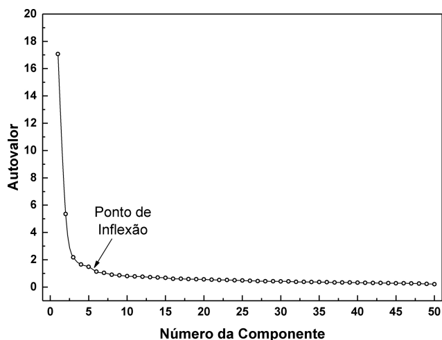
Figura 1: Scree plot obtido através da aplicação da AFE utilizando a versão completa do EMADF (com 50 itens). A seta mostra o ponto de inflexão do gráfico utilizado para definir o número de fatores a serem mantidos de acordo com o scree test .
