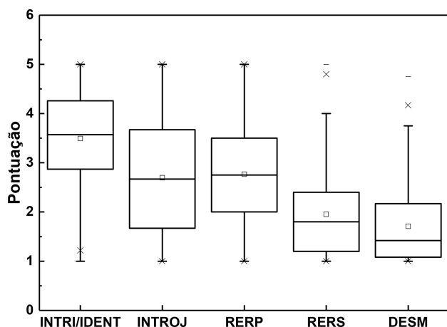
Figura 2: Pontuação atribuída a cada um dos fatores identificados na AFE considerando a versão completa do EMADF (com 50 itens).
