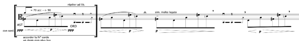
FIGURA 1 – Prologue (GRISEY, 1976, p.1, Linha 1). Destaque para a scordatura da viola, com a corda IV afinada em Si (e que permanece válida para todos os próximos exemplos da peça).
