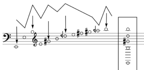
FIGURA 7 –Parciais de trombone a partir de Mi grave e curva de distribuição de energia dos parciais, realçando parciais ímpares. Os parciais mais salientes são aqueles empregados por Grisey para os primeiras neumas de Prologue . 19
