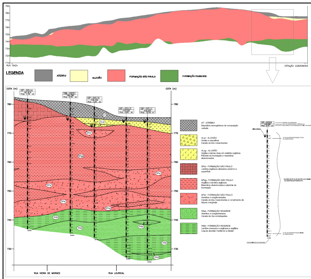
Figura 5 – Seção geológica esquemática ao longo da Av. Washington Luís.
