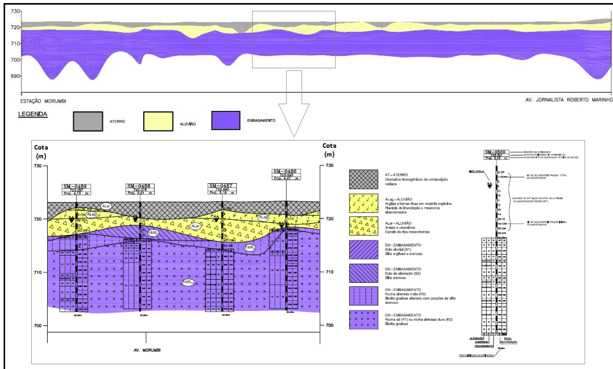
Figura 3 – Seção geológica esquemática ao longo da Marginal Pinheiros entre a Estação Morumbi e a Av. Jornalista Roberto Marinho. Detalhe: Seção geológico-geotécnica próxima ao cruzamento da Av. das Nações Unidas com a Av. Morumbi.
