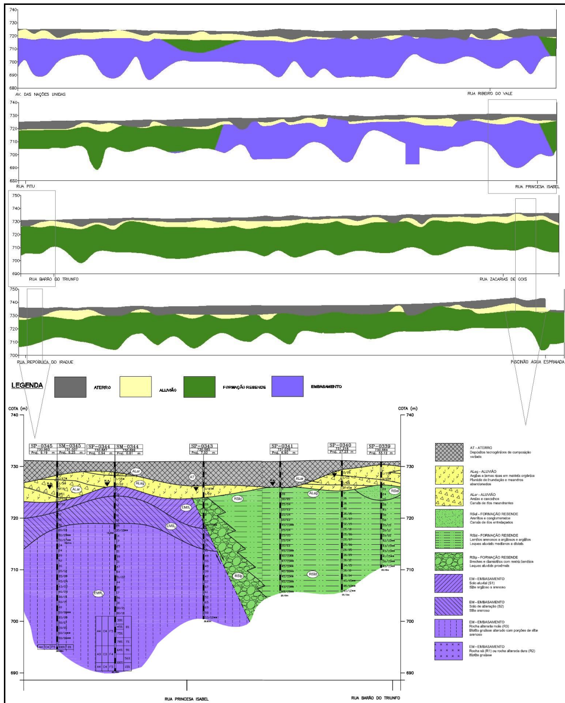
Figura 4 – Seção geológica esquemática ao longo da Av. Jornalista Roberto Marinho entre o cruzamento com a Av. das Nações Unidas e o enlace próximo a Av. Washington Luís (Piscinão Água Espreada).
