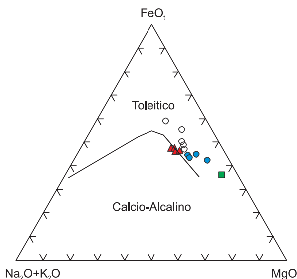
FIGURA 3. Diagrama AFM ( \text{Na}_2\text{O}+\text{K}_2\text{O} )- \text{FeO} - \text{MgO} para classificação geral dos litotipos máficos-ultramáficos, segundo proposta de Irvine & Baragar (1971). Símbolos: triângulos = diabásios; círculo vazio = gabros; círculos preenchidos = hornblenda gabros e quadrados = piroxênio hornblendito.
