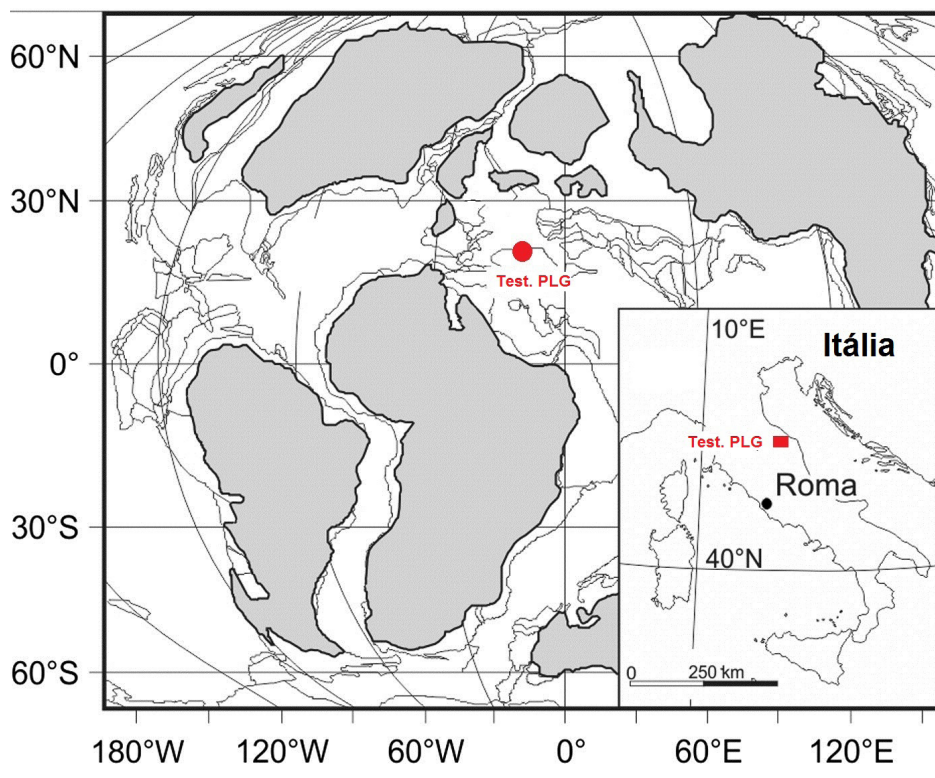
Figura 1 - Reconstrução paleogeográfica para aproximadamente 125 Ma modificada de Huber e Leckie (2011) mostrando a localização do testemunho PLG, Itália.
