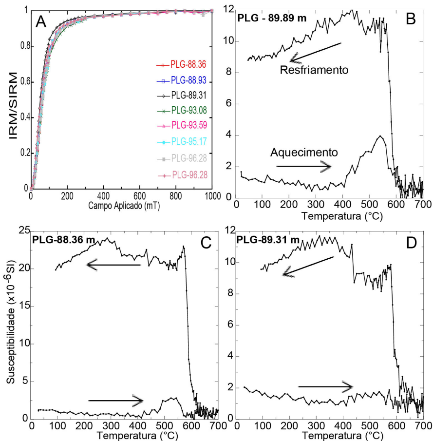
Figura 3 – (A) Curvas MRI para 8 amostras representativas do intervalo estudado. (B, C, e D) Curvas termomagnéticas de 3 amostras do intervalo estudado. Ambas técnicas indicam a magnetita como portador magnético principal.
